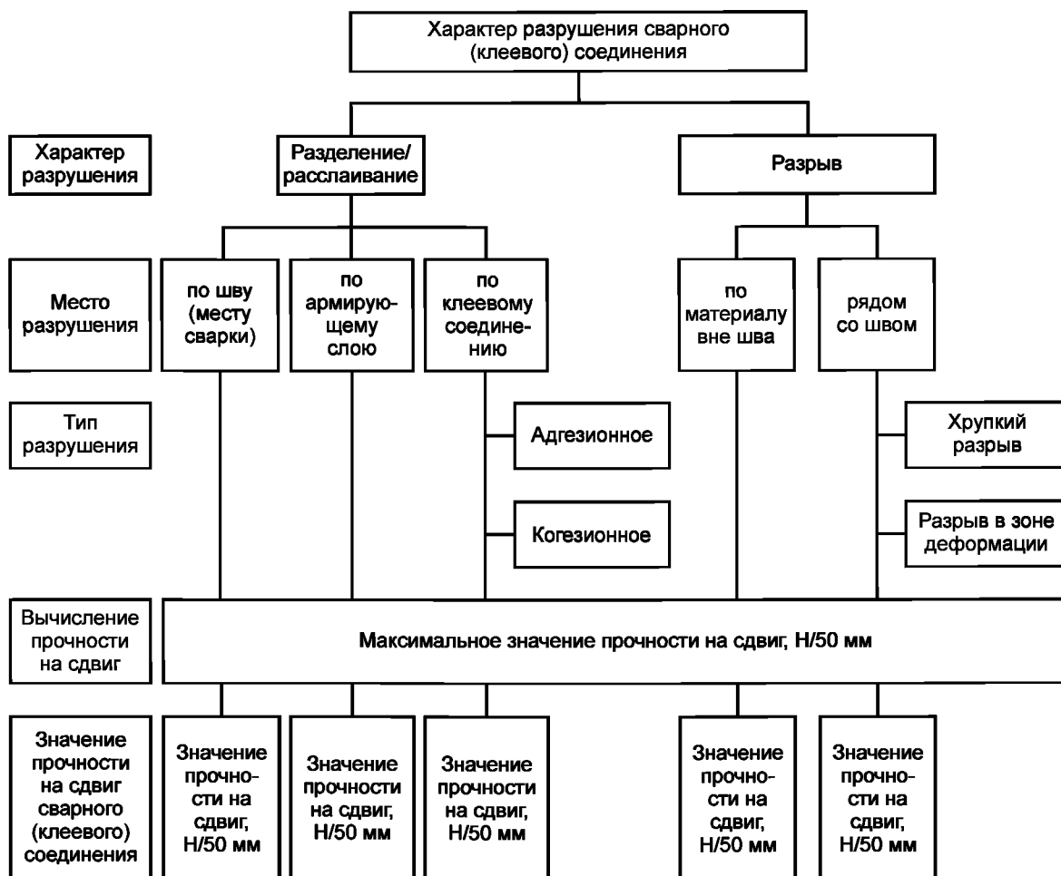
Рисунок А.1 — Характер разрушения сварного (клеевого) соединения
