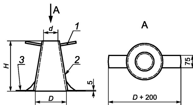
Рисунок А.1 — Конус для определения подвижности
