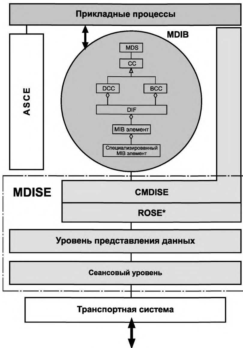
Рисунок 1 – Стек MDC
