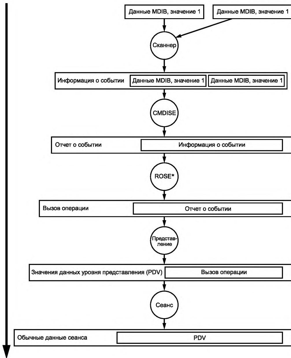
Рисунок 2 — Поток данных, проходящий через коммуникационный стек
