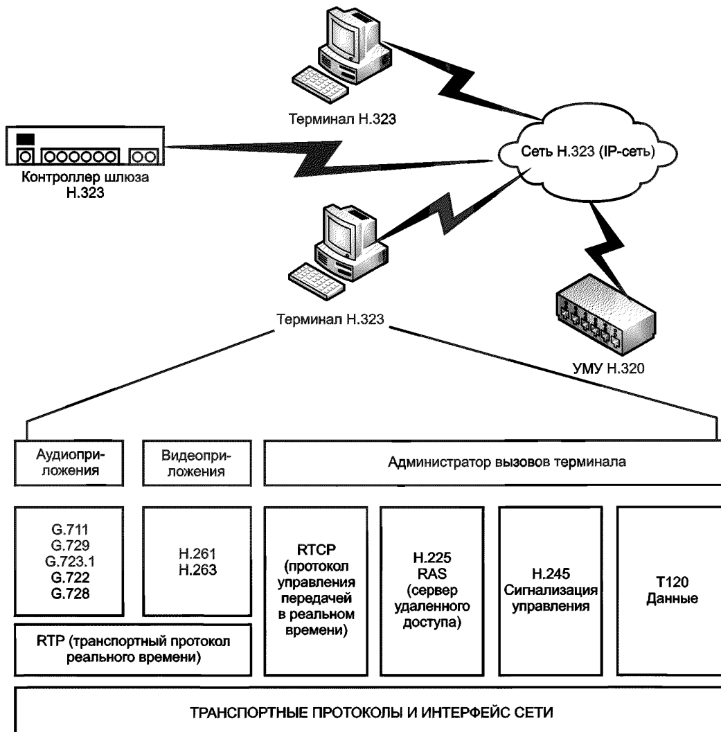
Рисунок 13 — Интероперабельность H.323
