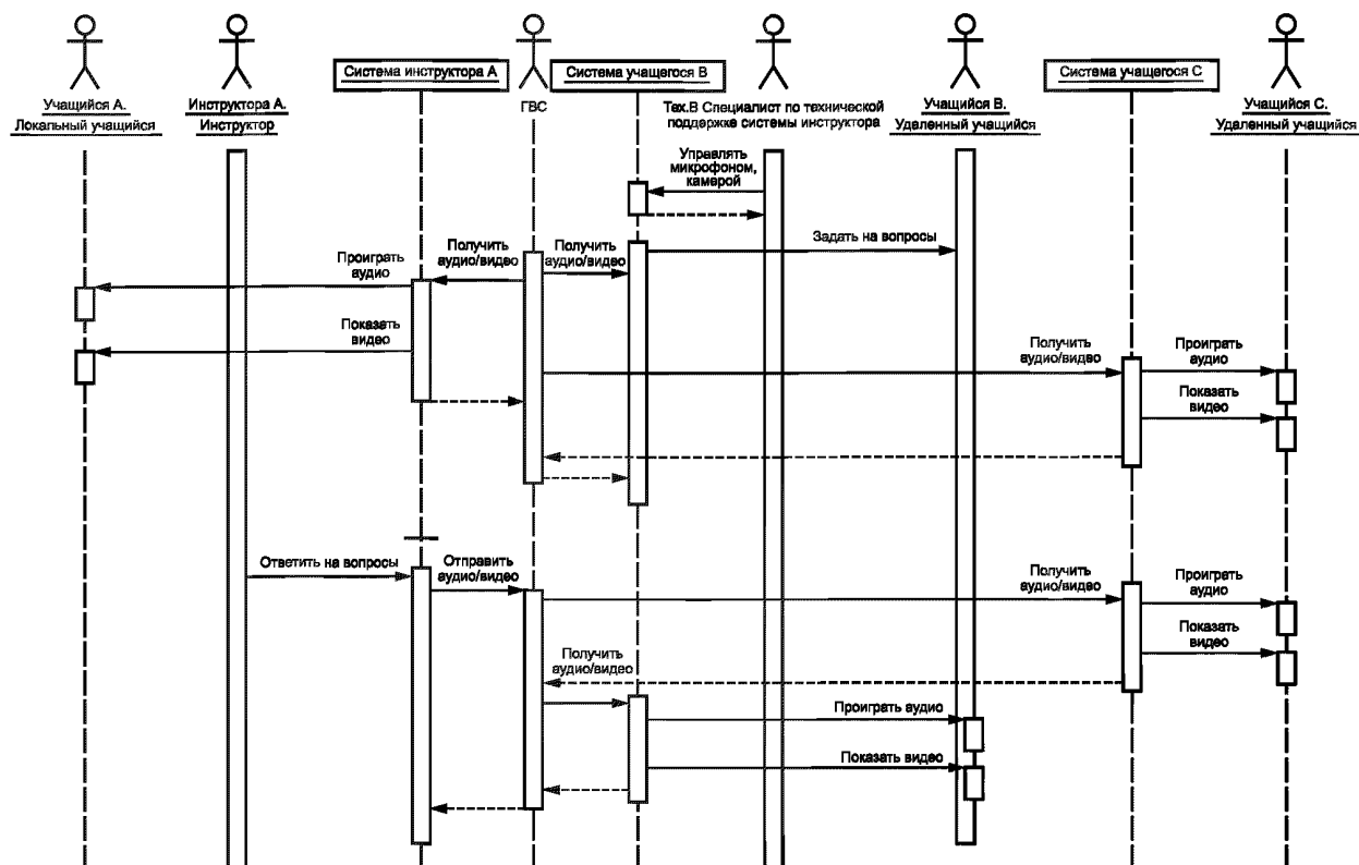
Рисунок 16 — Взаимодействие во время сессии в форме «Вопрос-ответ»
