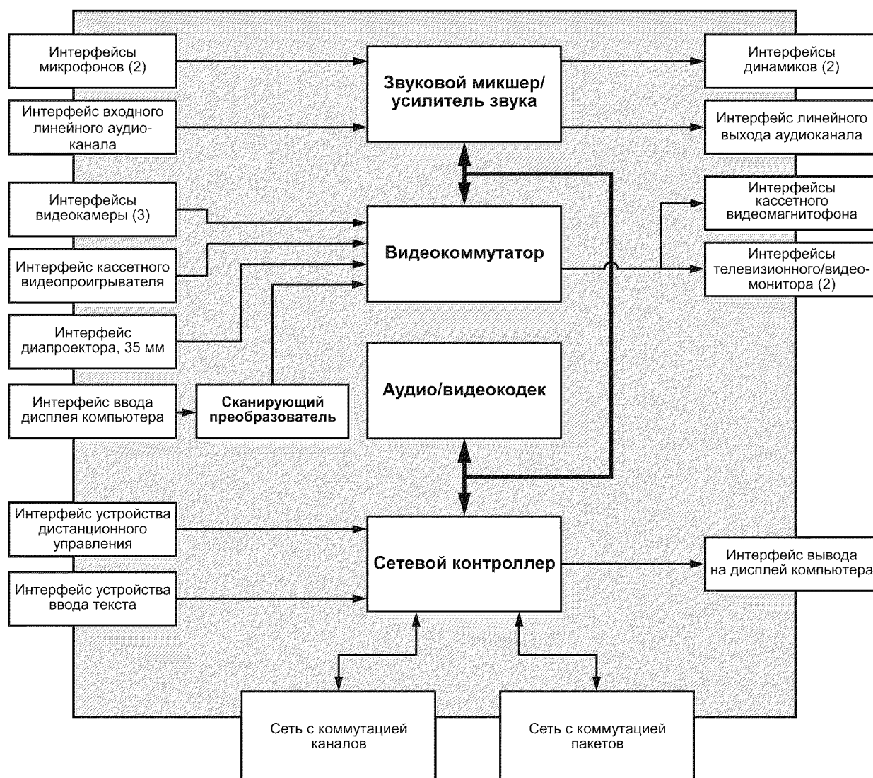
Рисунок 9 — Содержание коммуникационного контроллера системы инструктора
