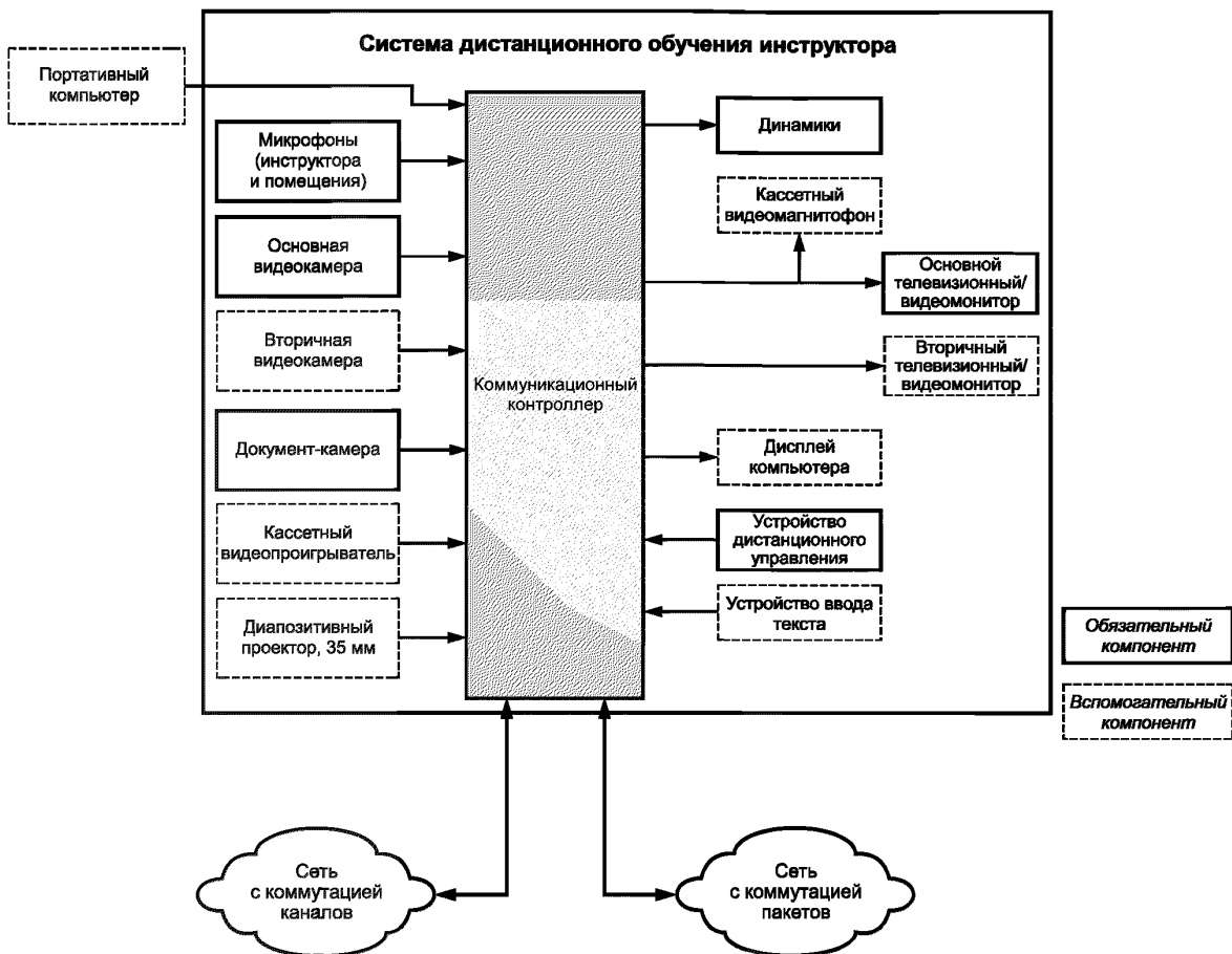
Рисунок 8 — Содержательная схема системы дистанционного обучения инструктора
