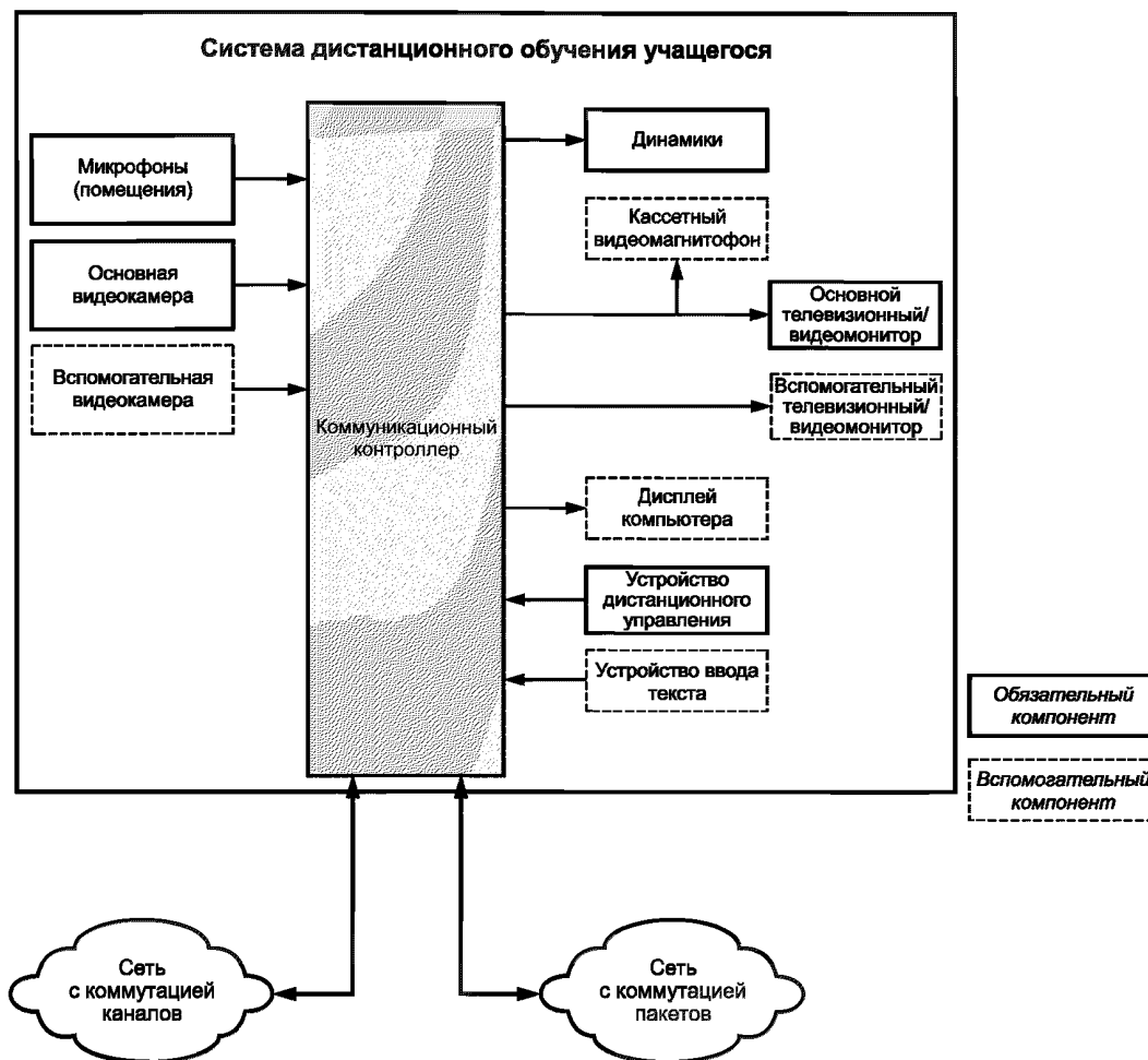
Рисунок 10 — Содержательная схема системы дистанционного обучения учащегося
