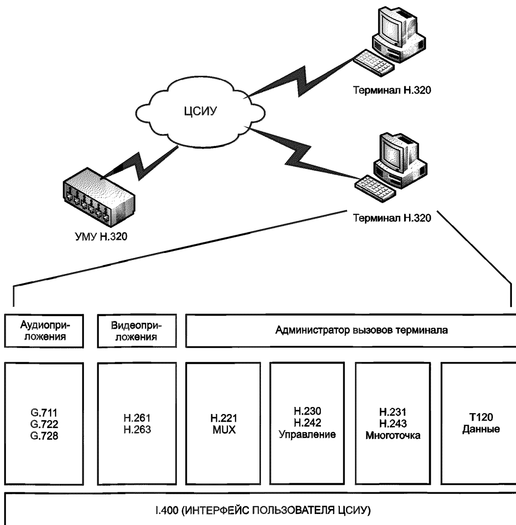
Рисунок 12 — Интероперабельность H.320
