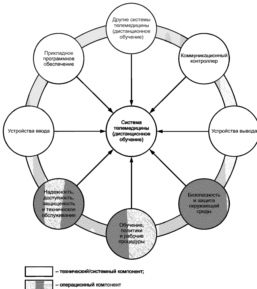
Рисунок 7 — Эталонная архитектура телемедицины
