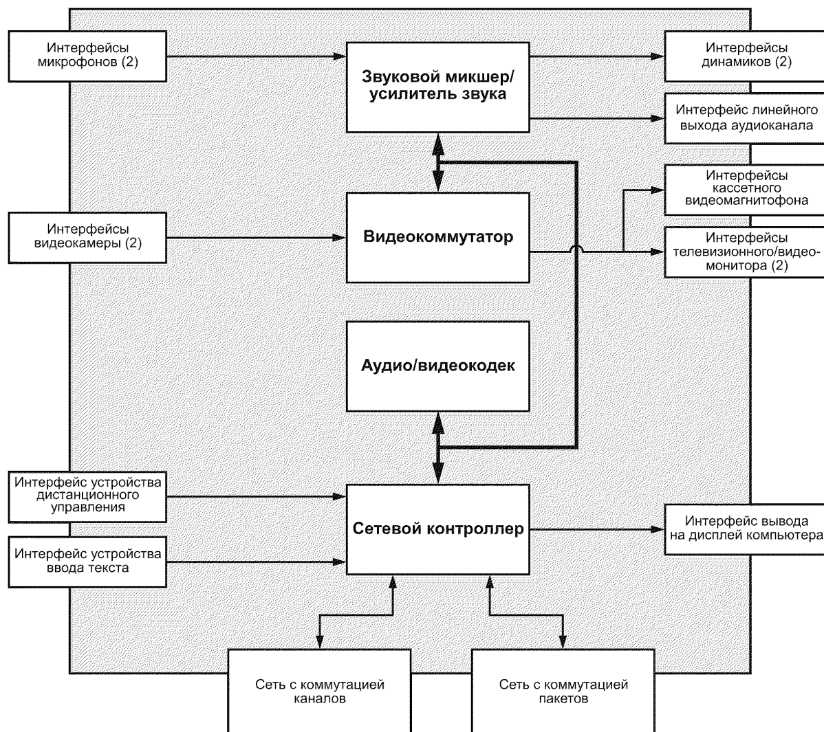
Рисунок 11 — Содержание коммуникационного контроллера связи системы учащегося
