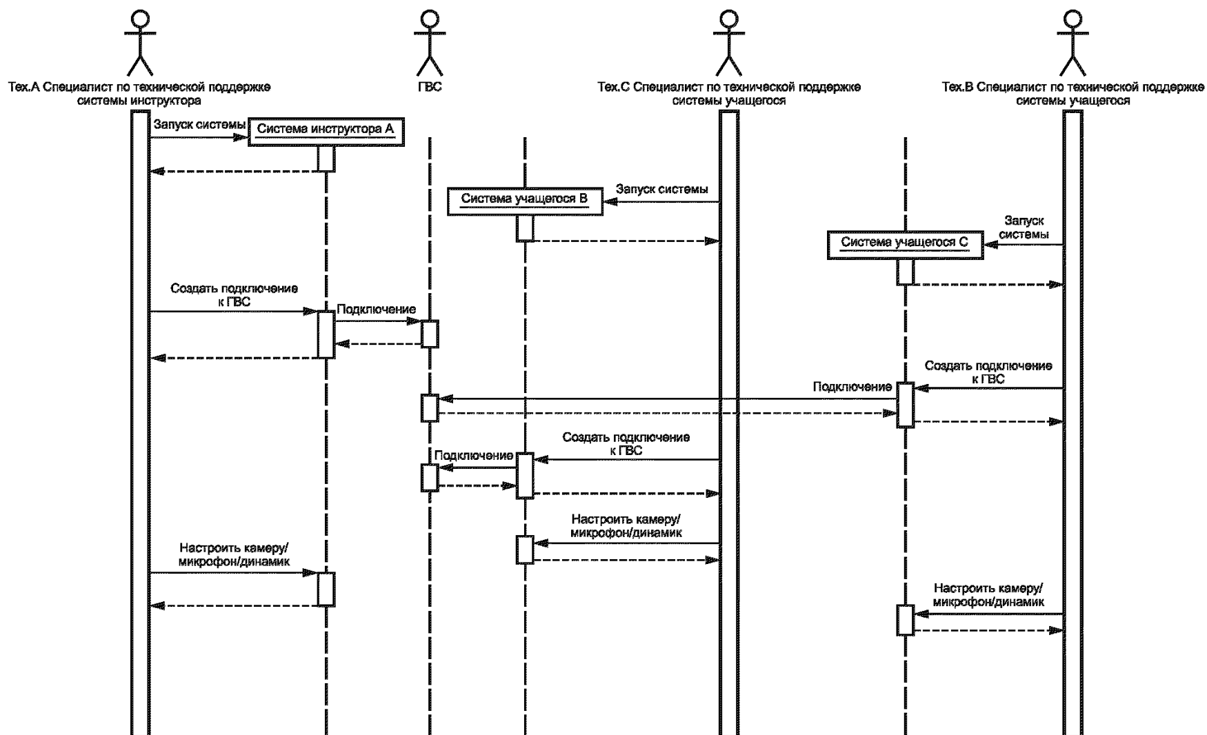
Рисунок 14 — Взаимодействия при запуске системы
