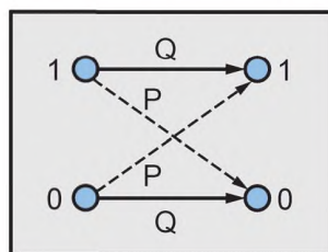
Рисунок В.2 — Двоичный симметричный канал (BSC)
