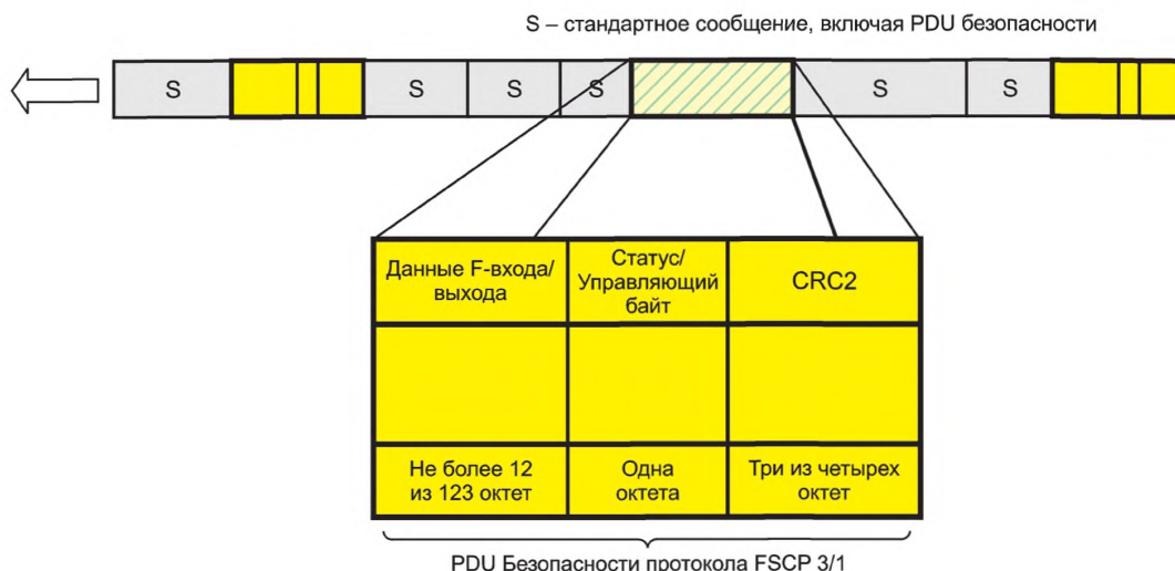
Рисунок 10 — Структура PDU безопасности профиля FSCP 3/1
