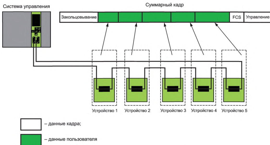
Рисунок 12 — Входные условия для коммуникации FSCP 6/7
