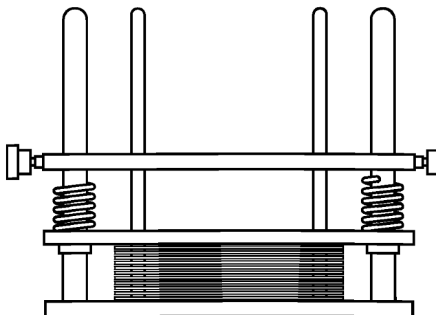
Рисунок 1 — Горизонтальное размещение
