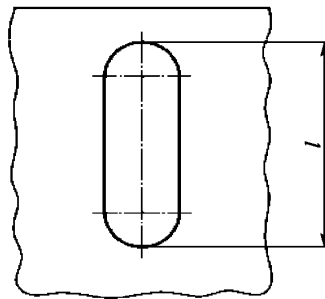
Угловой шов в продольном отверстии
