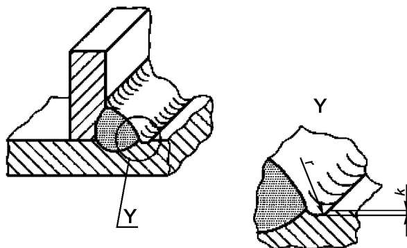
Рисунок 17 — Улучшение границы сварного шва
