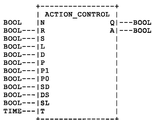
а) С логикой «завершающего сканирования»
