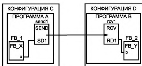
с) Функциональные блоки взаимодействия
