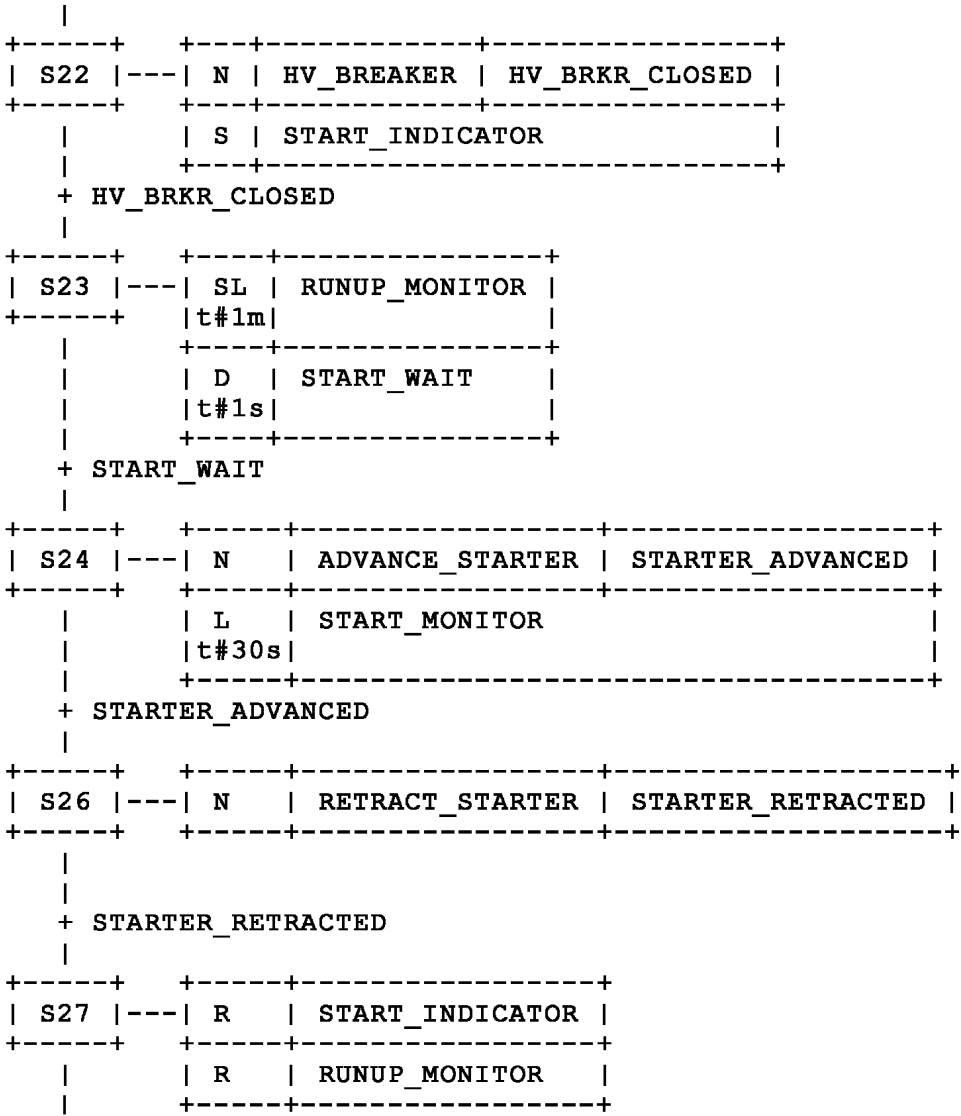
а) Представление SFC
