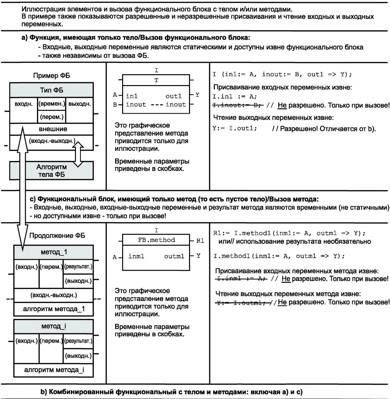
Рисунок 20 — Функциональный блок с необязательным телом и методами (иллюстрация)
