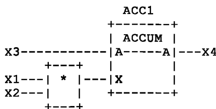
д) Допустимое использование экземпляра функционального блока
