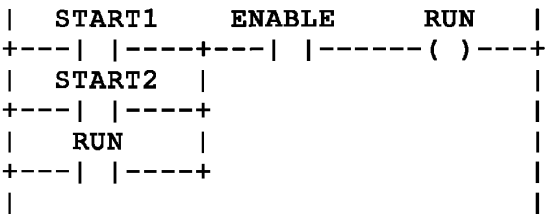
с) Эквивалент в языке LD
