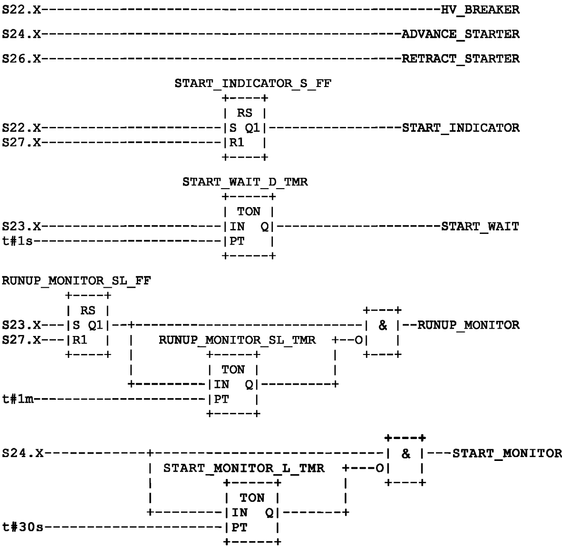
б) Функциональный эквивалент Примечание — В данном примере не показана полная сеть SFC и ее соответствующие объявления.
