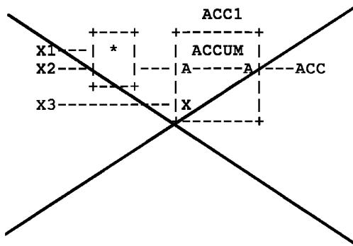
е) Неразрешенное использование экземпляра FB
