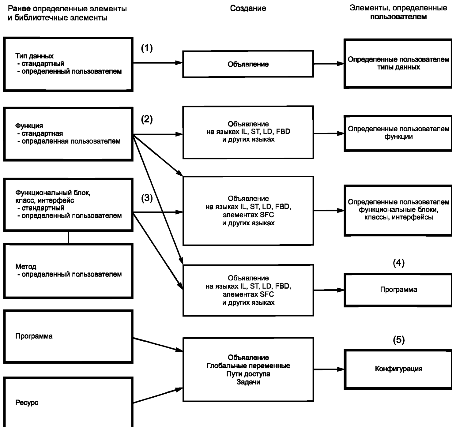
Рисунок 3 — Сочетание элементов языка программируемых контроллеров, лист 1
