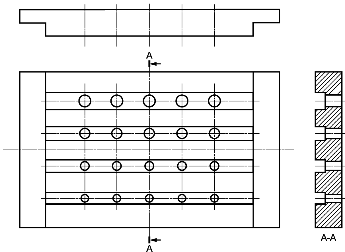
б) Стальная плита нагрузателя
