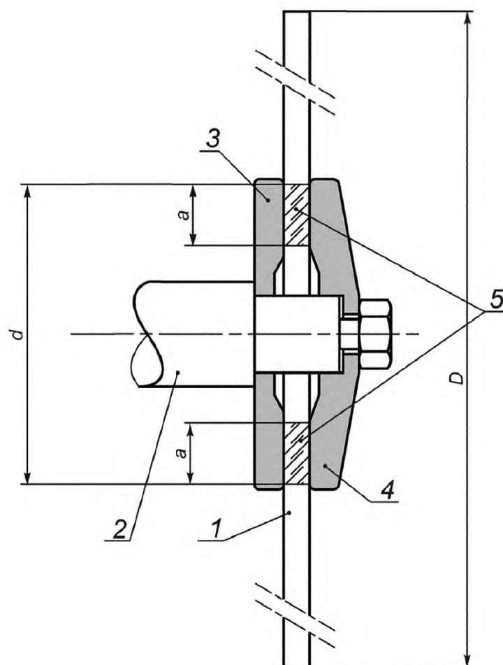
1 — пильный диск; 2 — инструментальный шпиндель; 3 — внутренний фланец; 4 — наружный фланец; 5 — зона перекрытия зажимных поверхностей; a — перекрытие зажимных поверхностей; D — максимальный назначенный диаметр пильного диска; d — наружный диаметр перекрытия зажимных поверхностей
