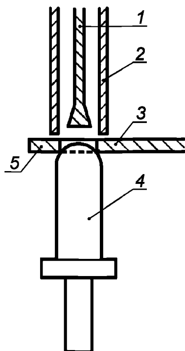
b) Врезная пила со свесом
