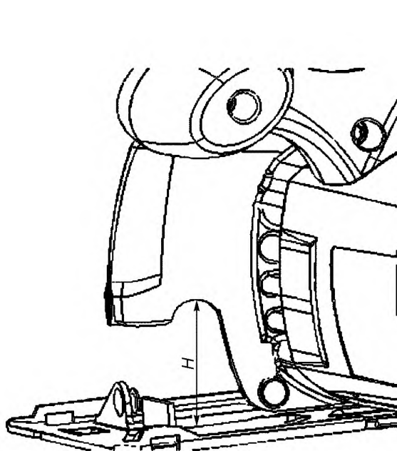
Рисунок 108а — Ограничение высоты проема (по 19.101.2.1). Высота проема для наблюдения
