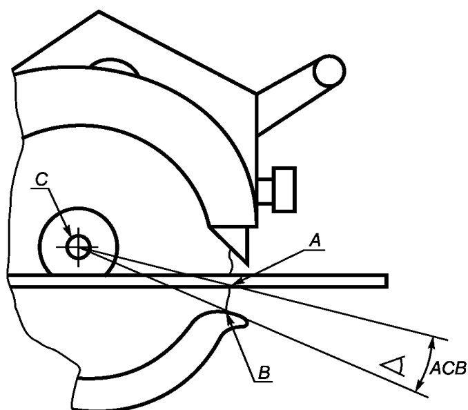
Рисунок 111 — Доступ к передней зоне зубчатого венца
