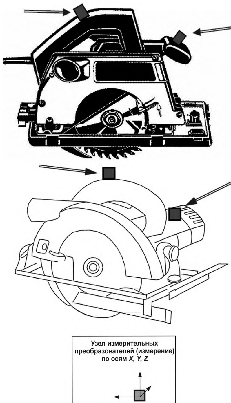
Рисунок I.101 — Положение измерительных преобразователей для дисковых пил
