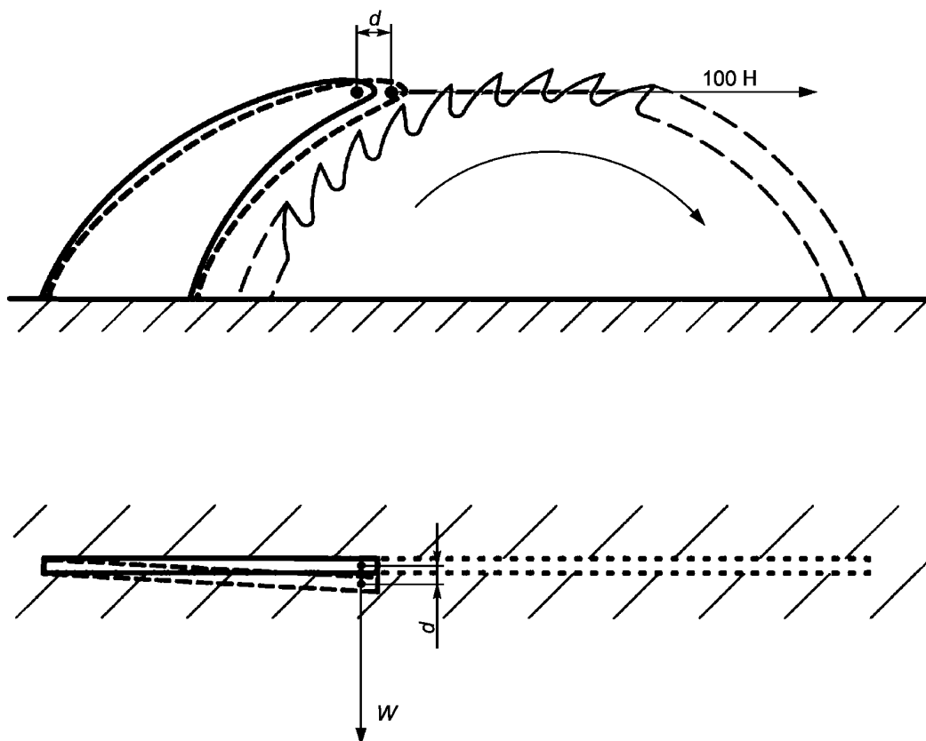
Рисунок АА.101 — Испытание устойчивости раскливающего ножа
