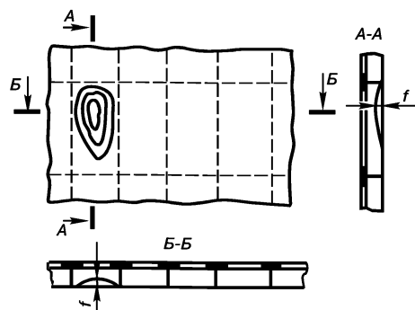
Рис. 3.4-2. Бухтина
