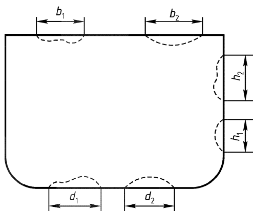
Рис 3.1.1. Вмятины корпуса
