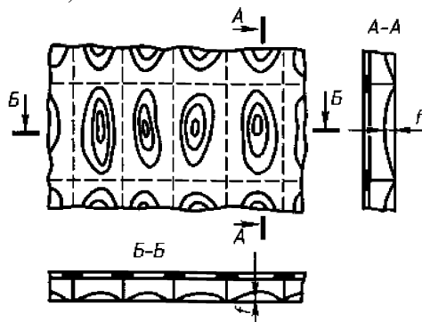
Рис. 3.4-1. Гофрировка
