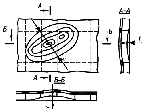
Рис. 3.4-3. Вмятина
