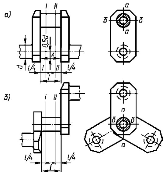
Рис. 2.1. Места определения износа шатунных ( а ) и коренных ( б ) шеек: А — место установки измерительного инструмента при определении раскеев
