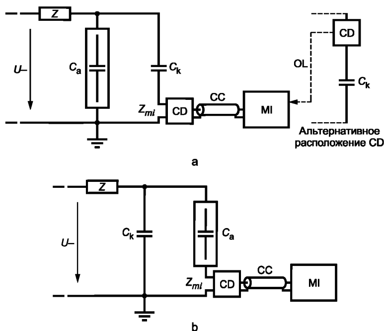
а — соединительное звено последовательно с соединительным конденсатором; б — соединительное звено последовательно с испытуемым объектом; U — высоковольтный источник; Z_{mi} — входное сопротивление измерительной системы; CC — соединительный кабель; OL — оптическая линия связи; C_a — испытуемый объект; C_k — соединительным конденсатором; CD — соединительное звено; MI — измерительный прибор; Z — фильтр
