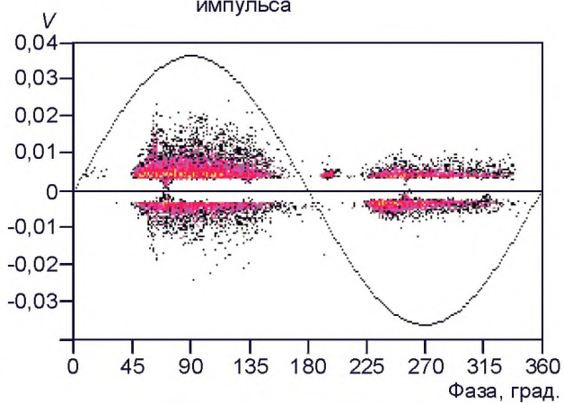
Рисунок D.5 — Пример выделения перекрестных помех
