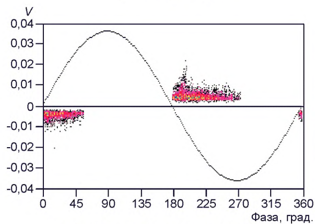
Рисунок D.5 — Пример выделения перекрестных помех
