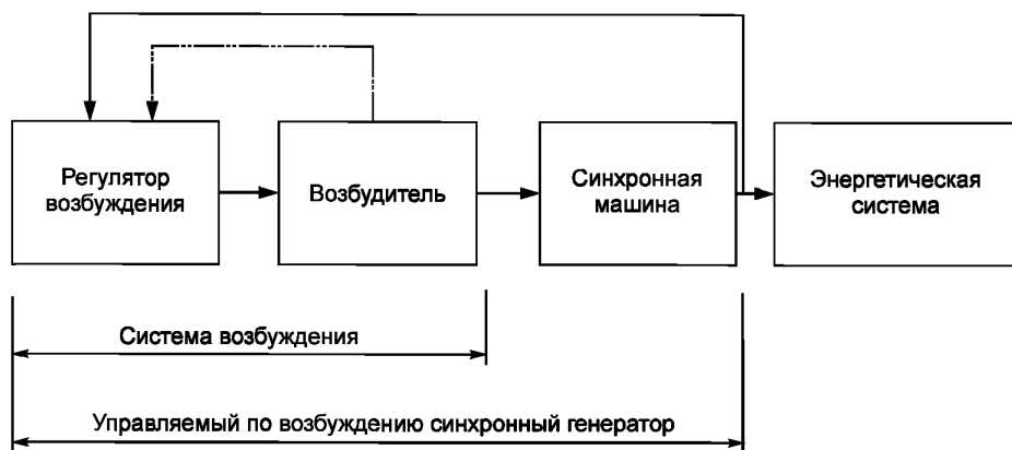
Рисунок 1 — Структура управляемого по возбуждению синхронного генератора
