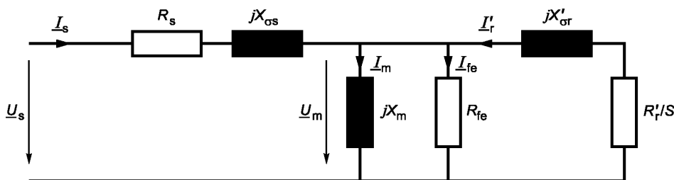
Рисунок 1 — Т-образная схема замещения
