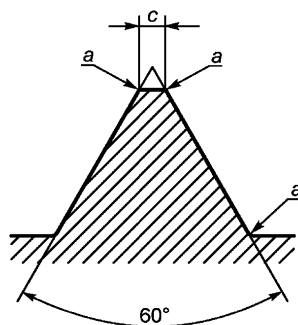
Профиль резьбы
