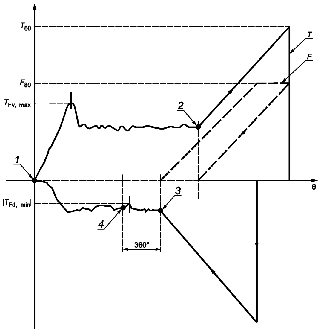
F — усилие предварительной затяжки; T — крутящий момент; \theta — угол поворота; 1 — точка, в которой впервые возникает стопорящий момент при закручивании и начинается измерение T_{Fv} ; 2 — точка посадки — окончание измерений T_{Fv} ; 3 — отсутствие контакта с испытательной пластиной/шайбой, начало измерения T_{Fd} ; 4 — окончание измерения T_{Fd}
