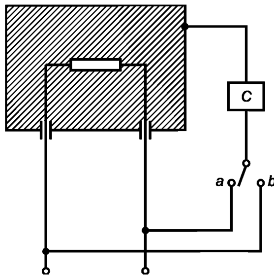
С — цепь из IEC 60990, рисунок 4
