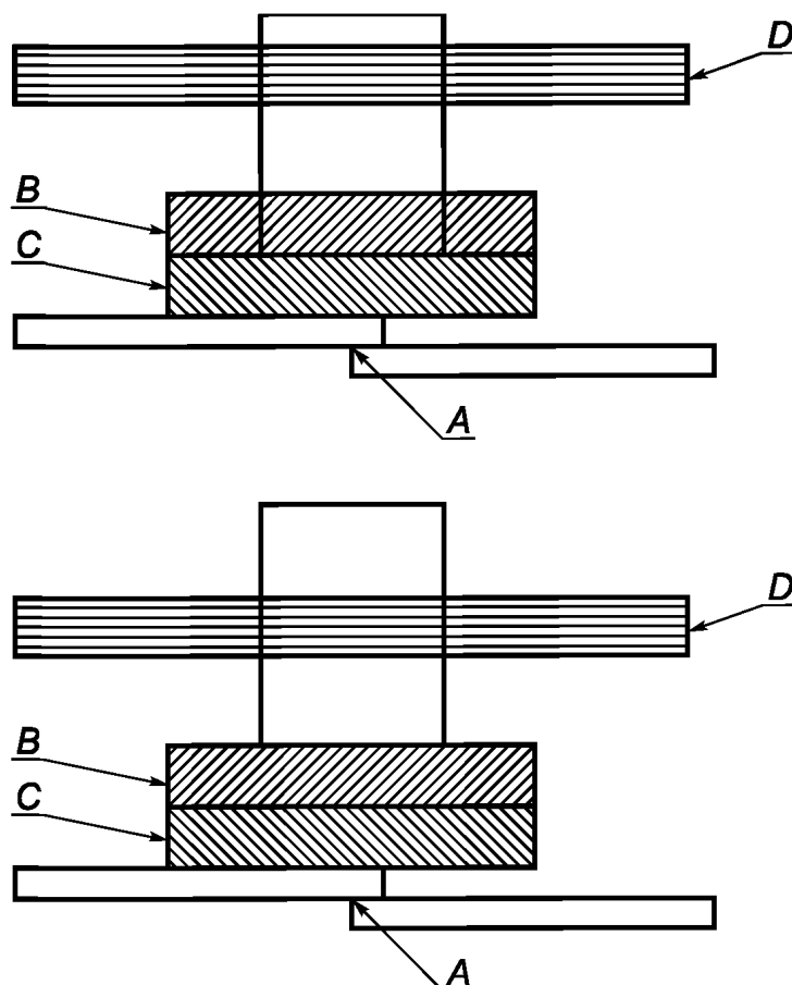
A — зона соединения; B, C и D — неметаллические материалы
