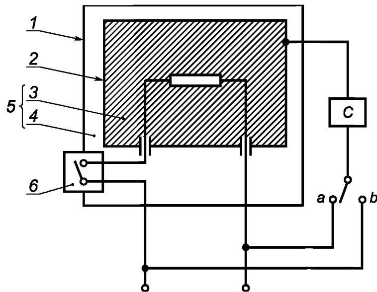
С — цепь из IEC 60990, рисунок 4; 1 — доступная часть; 2 — недоступная металлическая часть; 3 — основная изоляция; 4 — дополнительная изоляция; 5 — двойная изоляция; 6 — усиленная изоляция
