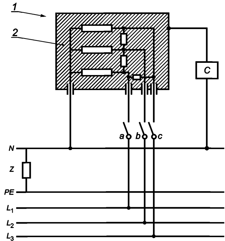
C — цепь из IEC 60990, рисунок 4; 1 — доступные части; 2 — основная изоляция; L_1, L_2, L_3, N — сеть питания с нейтралью; PE — провод защитного заземления; Z — высокий импеданс нейтраль-земля в системах IT
