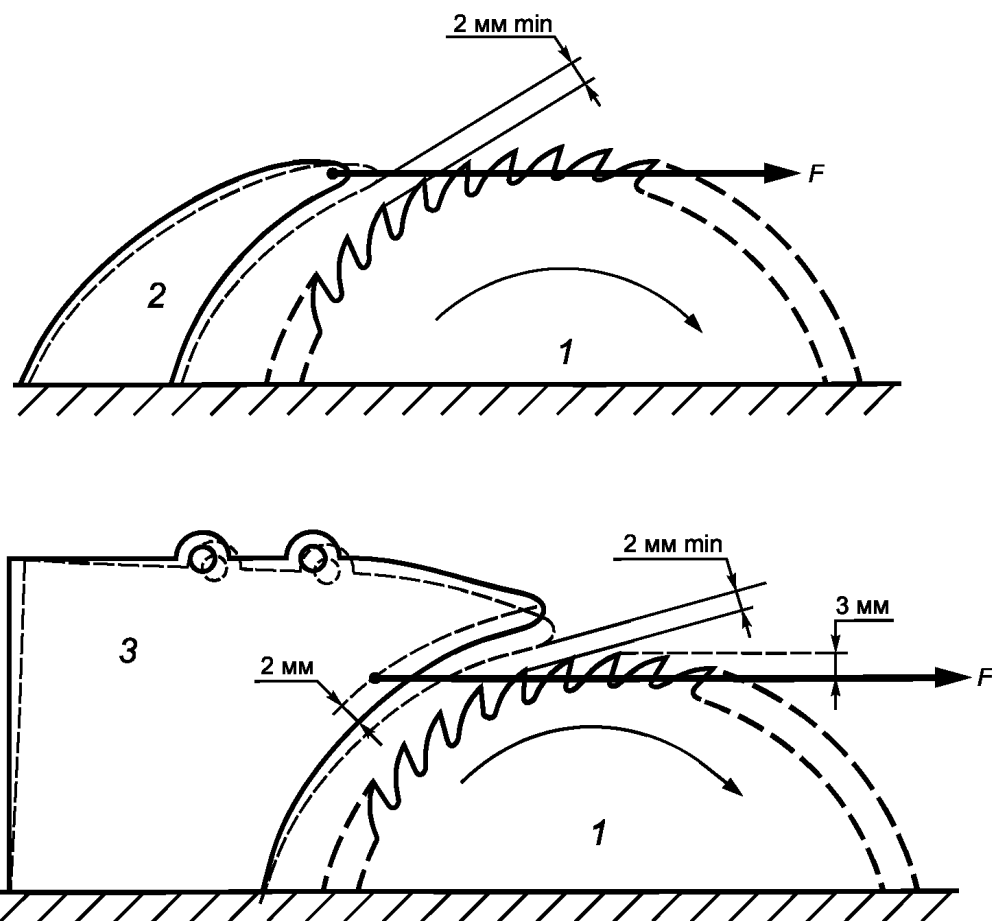
1 — пильный диск; 2 — расклинивающий нож; 3 — нерегулируемый или регулируемый удлиненный расклинивающий нож; F — тянущее усилие
