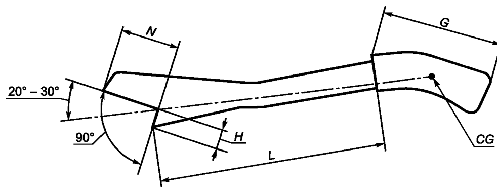
Рисунок 110 — Толкатель
