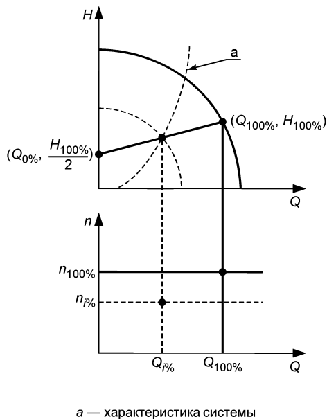
Рисунок 1 — Определение рабочей точки на режиме недогрузки
