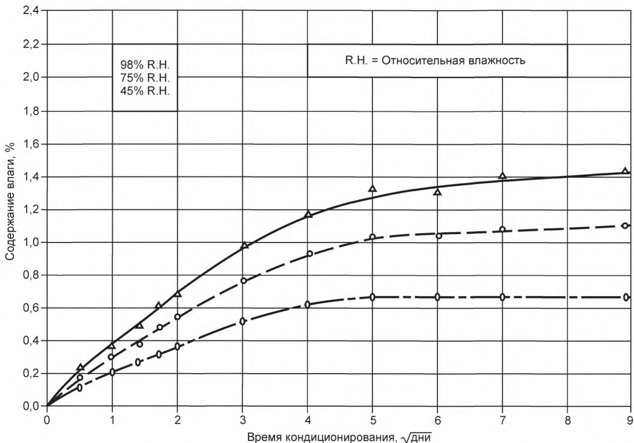
Рисунок 1 — Пример графика влагопоглощения углерод/эпоксидных (0,45—45,0) S слоистых материалов из восьми слоев при температуре 48,9 °C (8)
