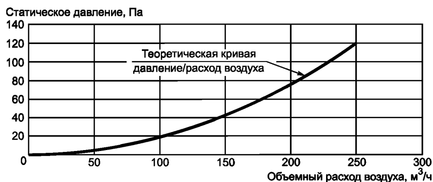
Рисунок В.1 — Кривая давление/объемный расход воздуха
