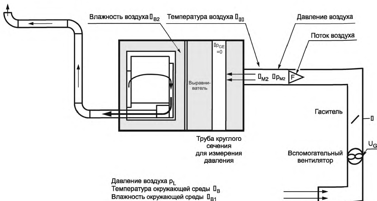
Рисунок Н.1 — Компоновка приемной камеры
