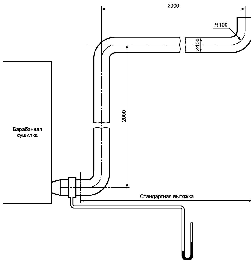
Рисунок В.2 — Стандартный вытяжной воздуховод
