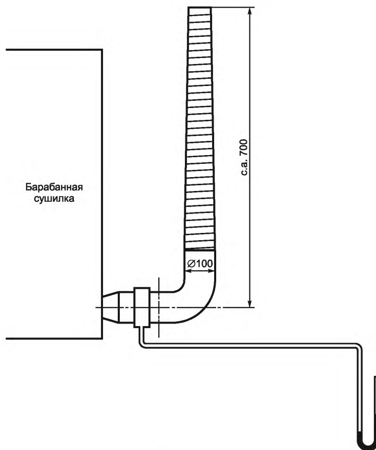
Рисунок В.3 — Стандартный вытяжной имитатор
