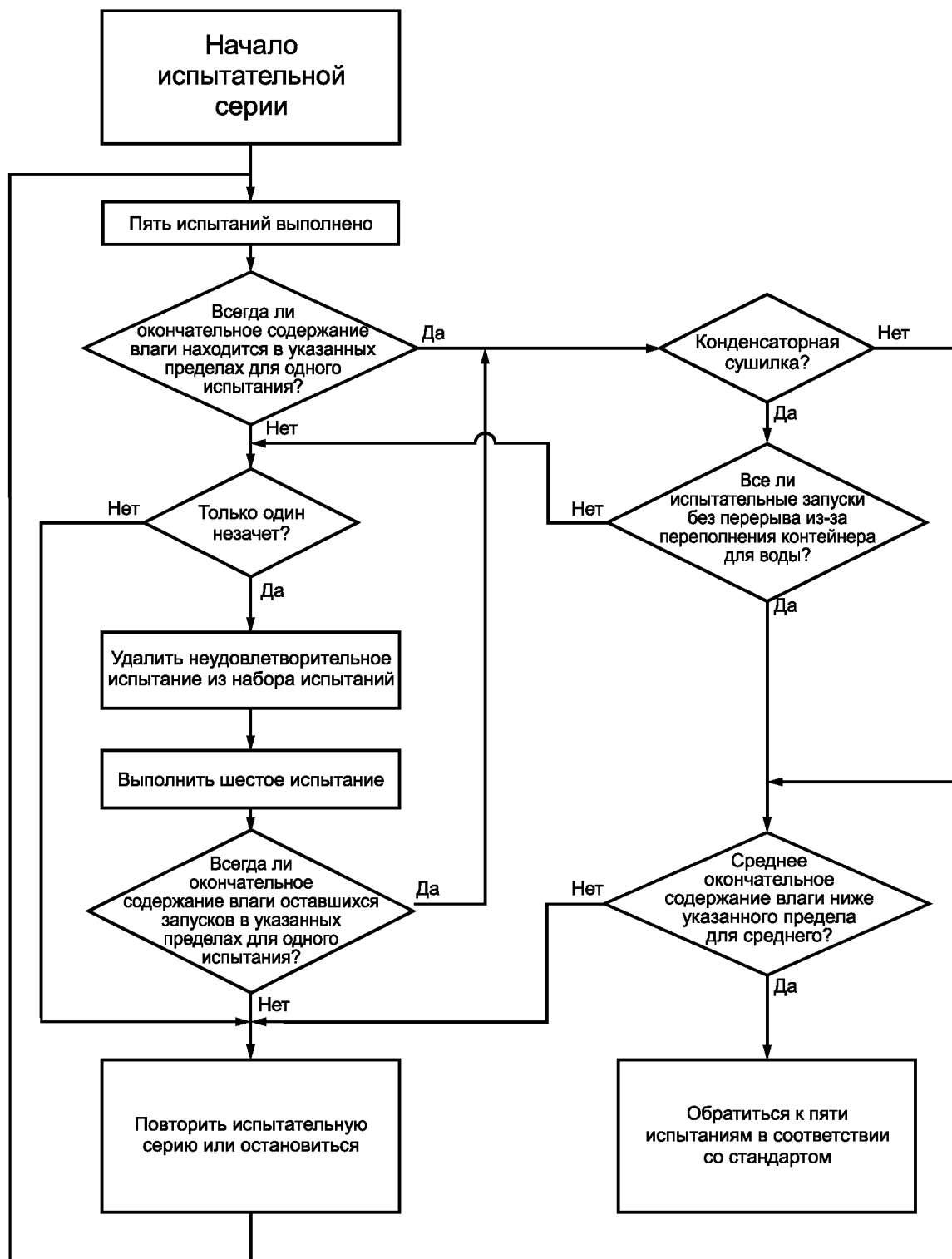
Рисунок С.2 — Схема принятия решений, иллюстрирующая требования для зачетной испытательной серии для неавтоматических барабанных сушилок
