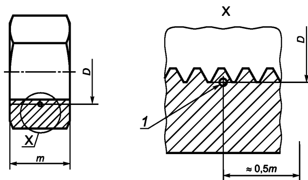
Рисунок 3 — Расположение точек измерения твердости на середине высоты гайки
