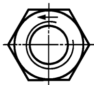
Рисунок 6 — Маркировка левой резьбы
