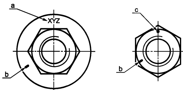
Рисунок 4 — Примеры символа маркировки
