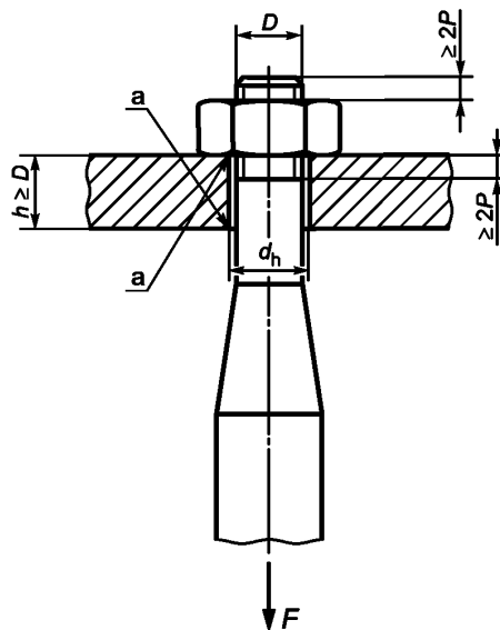
Рисунок 1 — Испытание на осевое растяжение
