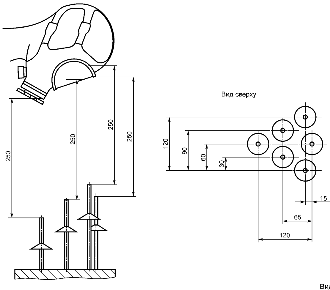
Рисунок 2 — Схема расположения шести горелок для проведения статического испытания устойчивости к воспламенению лицевой части СИЗОД с шестью горелками
