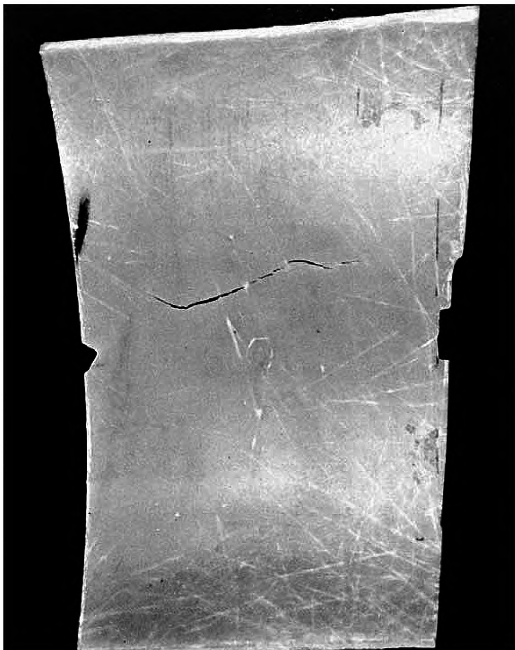
Рисунок А.15 — Трещина с избыточной смолой
