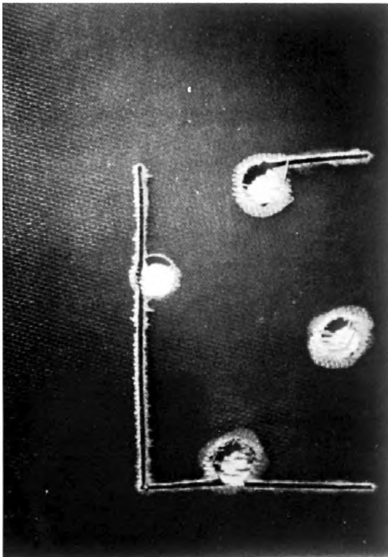
Рисунок А.3 — Расплаивание вследствие неправильной механической обработки
