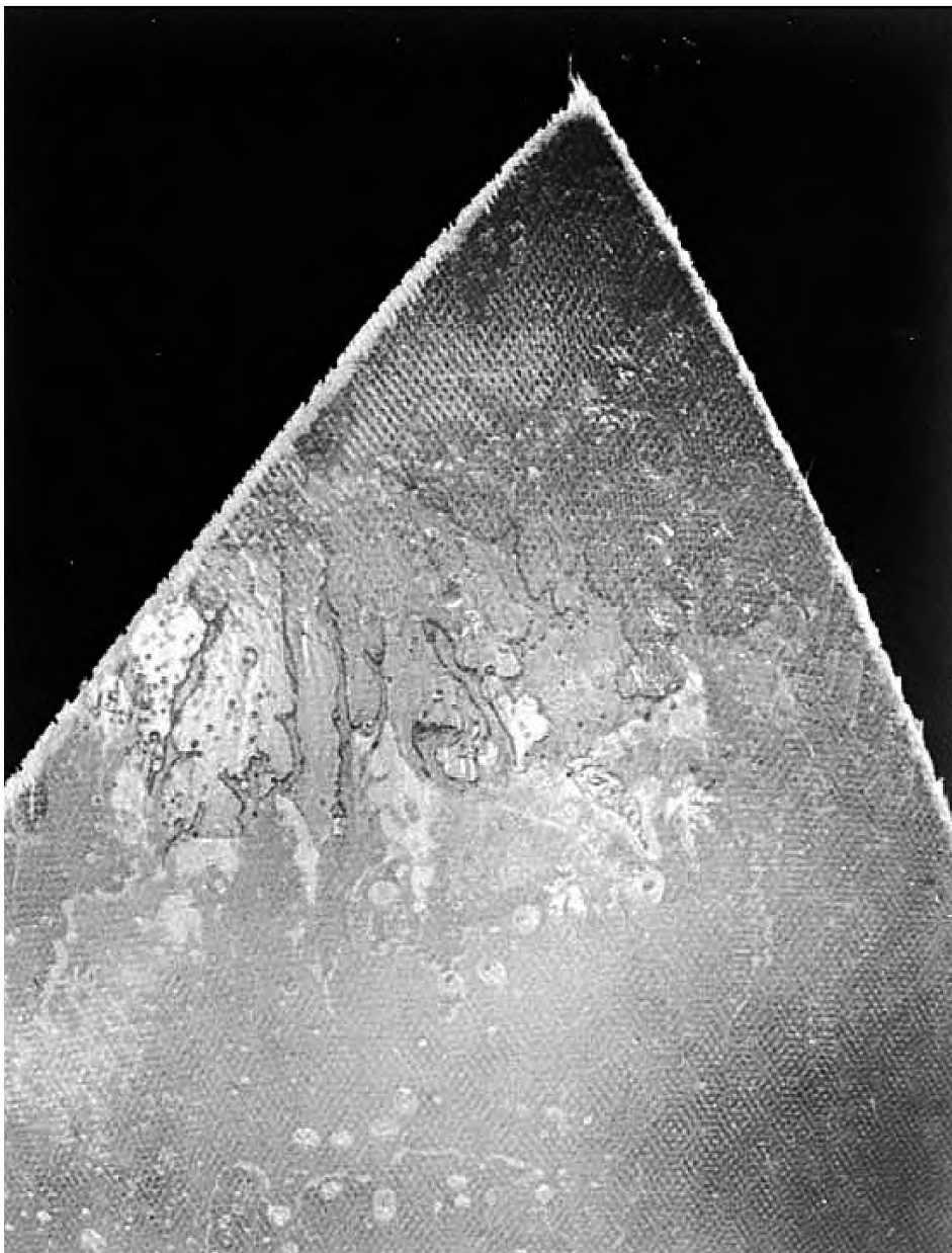
Рисунок А.14 — Смоляной карман
