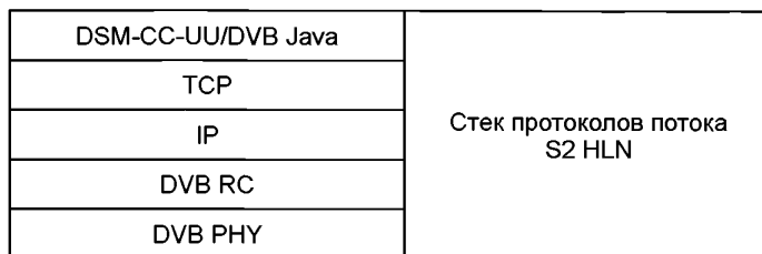
Рисунок 8 — Схема преобразования протоколов потока S2 HLN резидентного шлюза DVB
