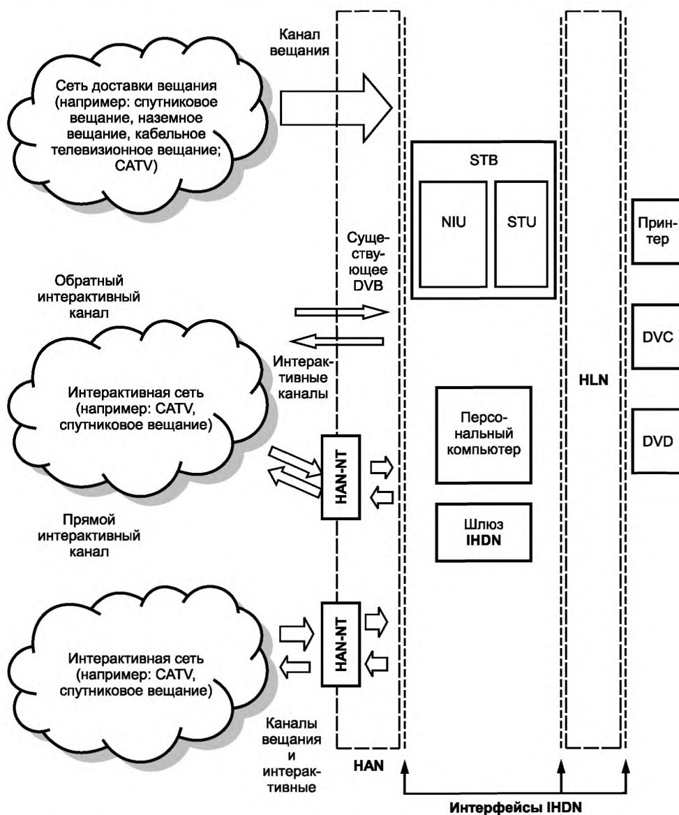
Рисунок 1 — Расширенная интерактивная эталонная модель системы DVB с IHDN
