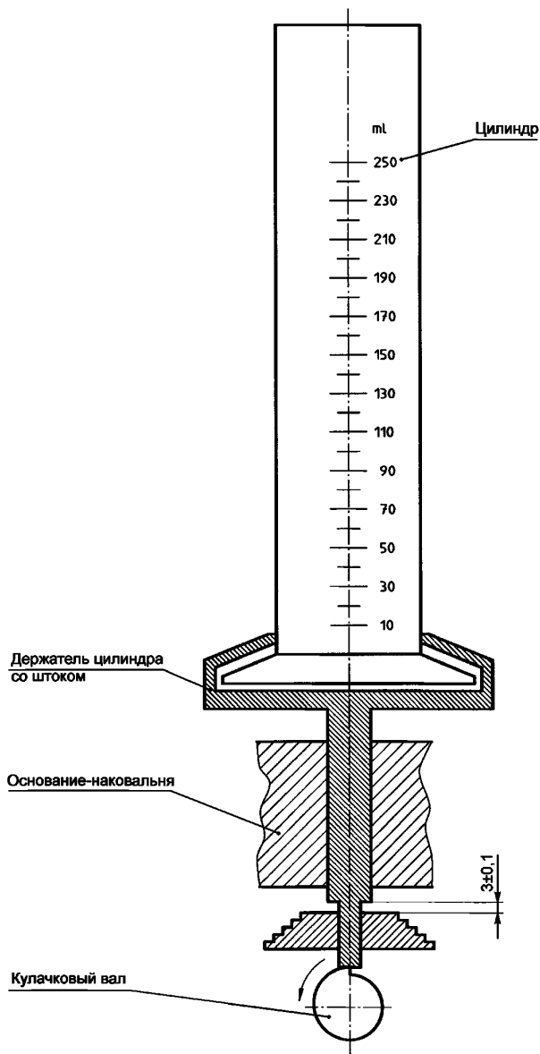
Рисунок 1 — Установка для измерения насыпной плотности кокса
