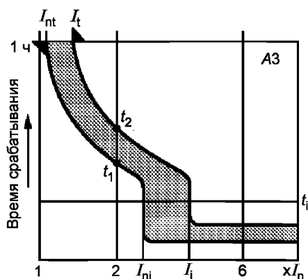
Рисунок А.3 — Характеристика тепловой и электромагнитной защиты
