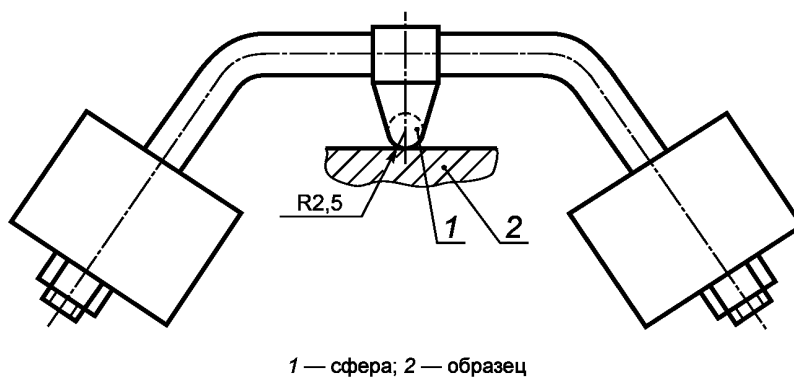
Рисунок 8 — Установка для испытаний давлением шарика
