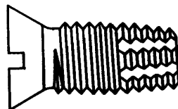
Рисунок 2 — Самонарезающий режущий винт
