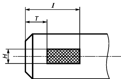
Рисунок Е.10 — Размеры штыревого наконечника
