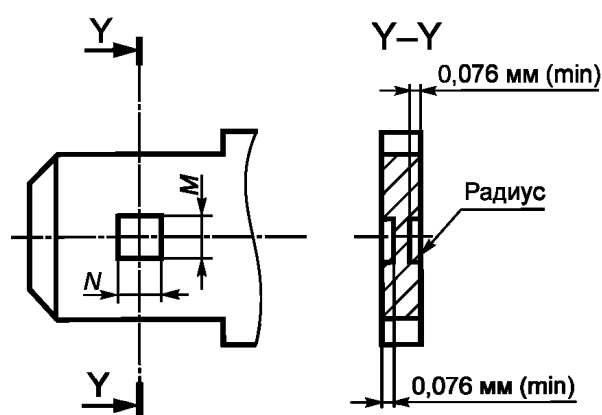
Рисунок Е.7 — Размеры круглых углублений фиксации (см. рисунок Е.6)
