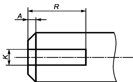
Рисунок Е.12 — Размеры штыревого наконечника
