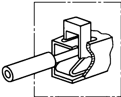
Рисунок Е.5 — Примеры безрезьбовых выводов
