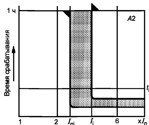
Рисунок А.2 — Характеристика только электромагнитной защиты
