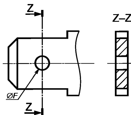
Рисунок Е.8 — Размеры прямоугольных элементов фиксации (см. рисунок Е.6)
