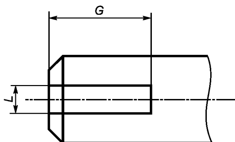
Рисунок Е.11 — Размеры штыревого наконечника
