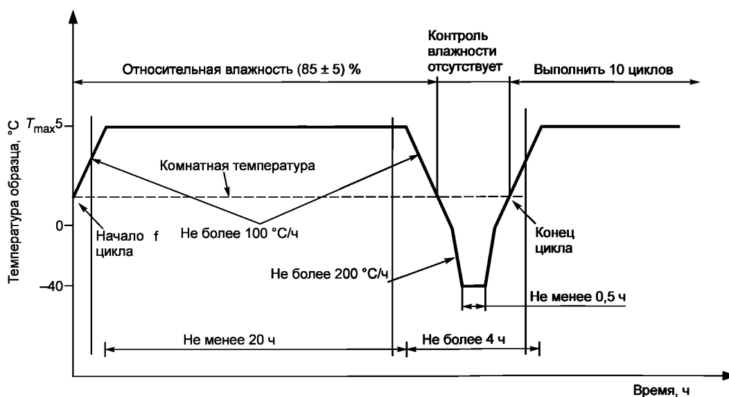
Рисунок 4 — Цикл термоциклирования при высокой влажности
