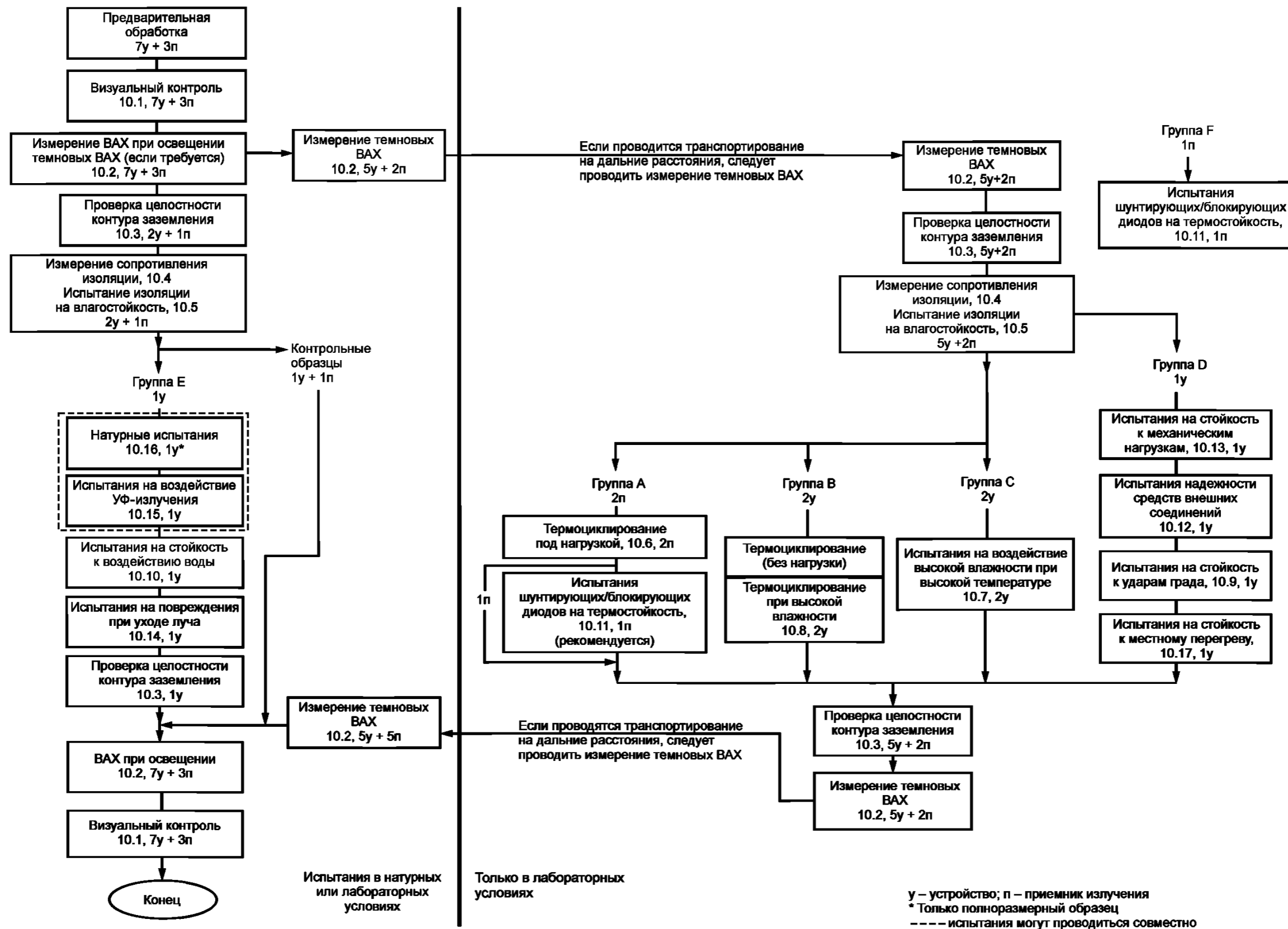
Рисунок 1 – Порядок проведения испытаний фотоэлектрических устройств с концентраторами, которые поставляются в готовом виде
