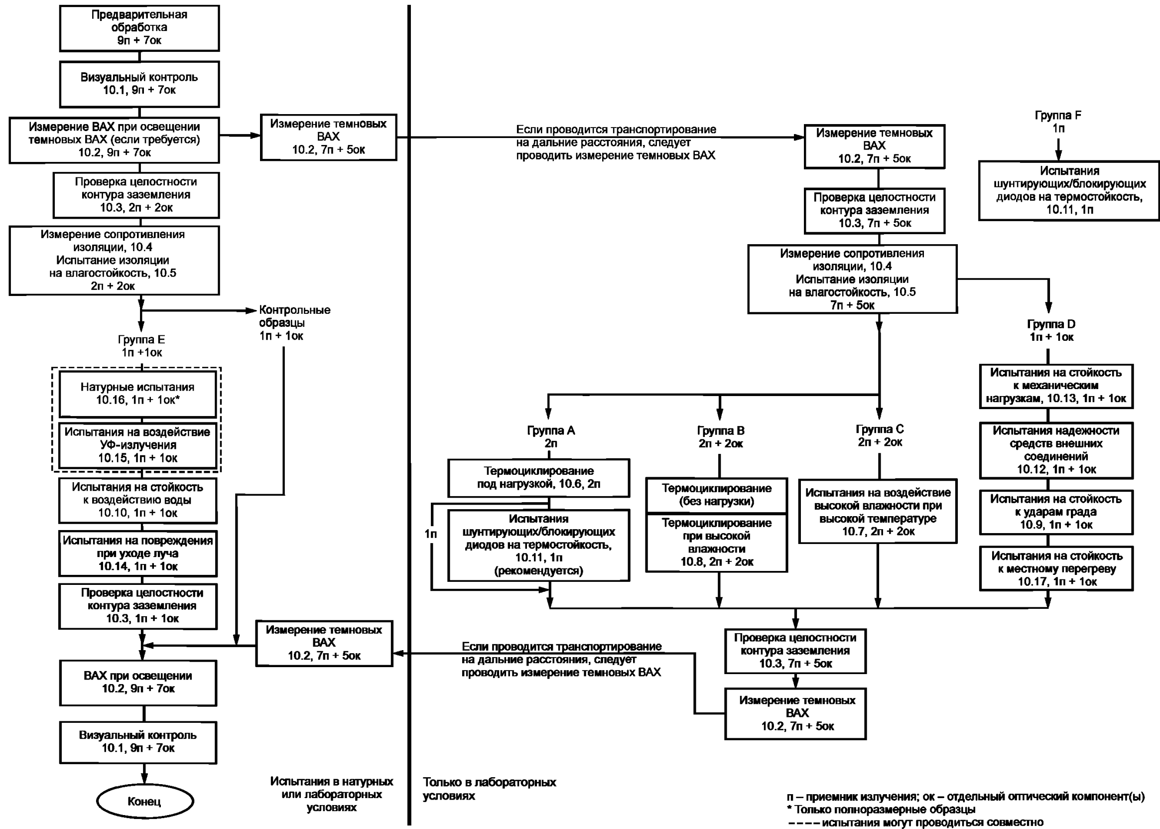
Рисунок 2 – Порядок проведения испытаний фотоэлектрических устройств с концентраторами, которые поставляются в разобранном виде и собираются на месте эксплуатации
