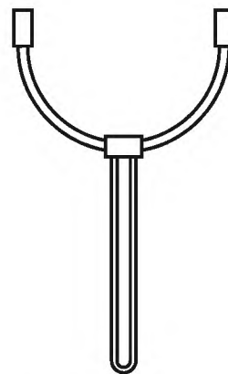
Рисунок 8 — Распорная деталь для центровки электрода
