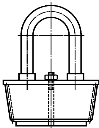
Рисунок 4 — Транспортировочный ниппель
