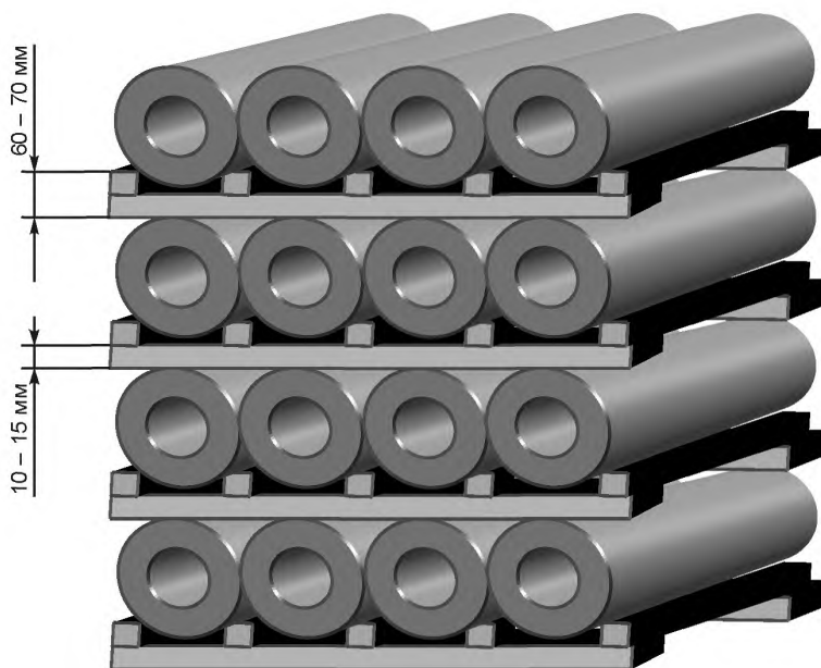
Рисунок 2 — Стеллаж для хранения электродов
