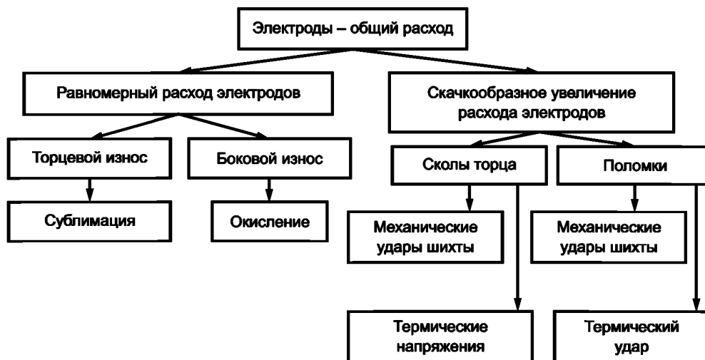
Рисунок 12 — Схема-модель процесса расхода электродов
