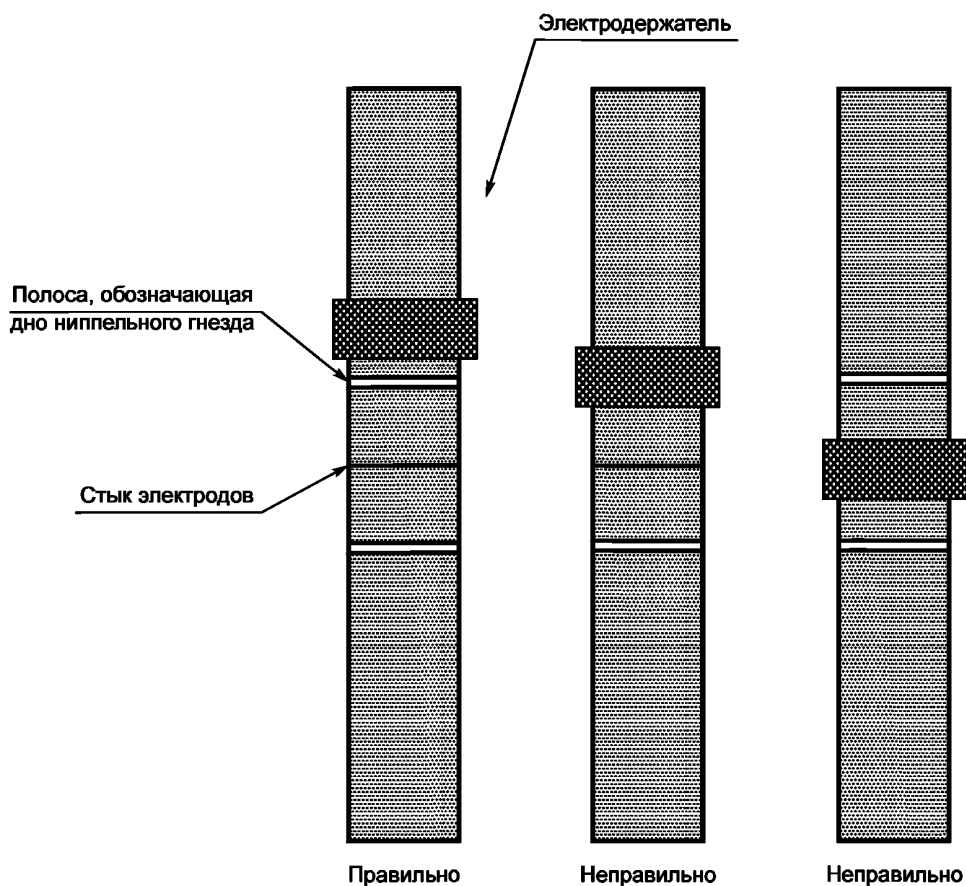
Рисунок 11 — Схема зажима электродов в электродержателе
