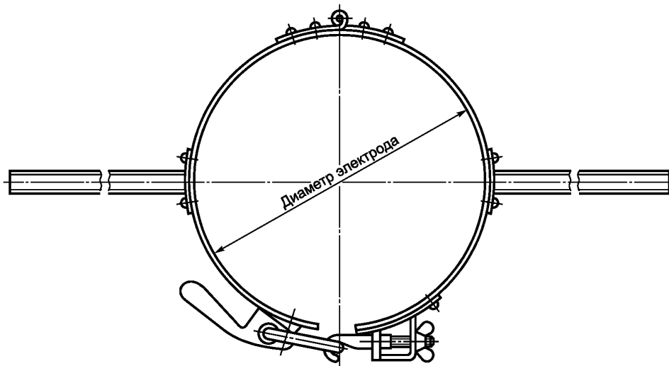
Рисунок 10 — Ручной зажим без ограничителя вращающего момента
