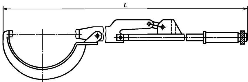
Рисунок 9 — Ручной зажим с ограничителем вращающего момента
