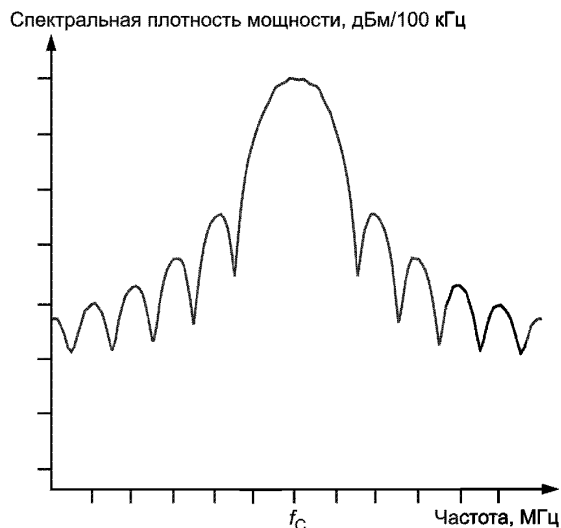
Рисунок 15 — Спектральная плотность мощности системы IEEE 802.15.4
