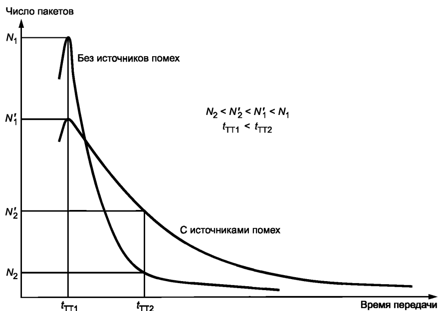
Рисунок 18 — Пример функций плотности распределения времени передачи
