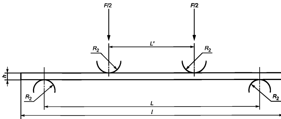
h — толщина образца, R_1 — радиус закругления пуансона, R_2 — радиус закругления краев опор, L — пролет между опорами, L' — пролет между верхними опорами, l — длина образца
