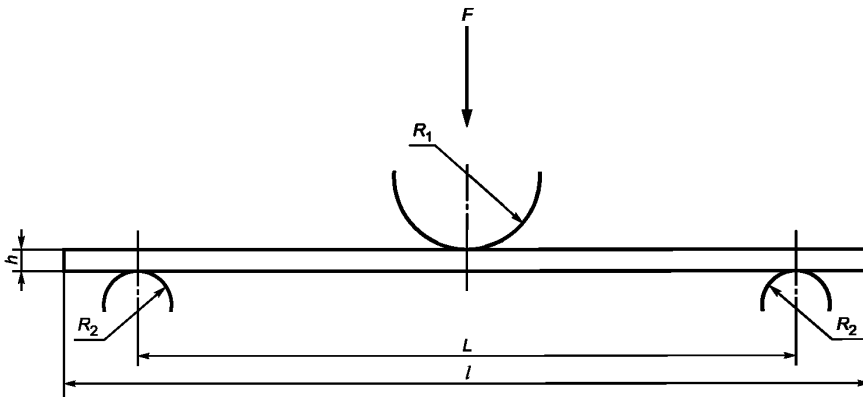
h — толщина образца, R_1 — радиус закругления пуансона, R_2 — радиус закругления краев опор, L — пролет между опорами, l — длина образца
