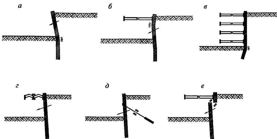
Рисунок 11.3 – Проектные ситуации, соответствующие разрушению конструктивных элементов
