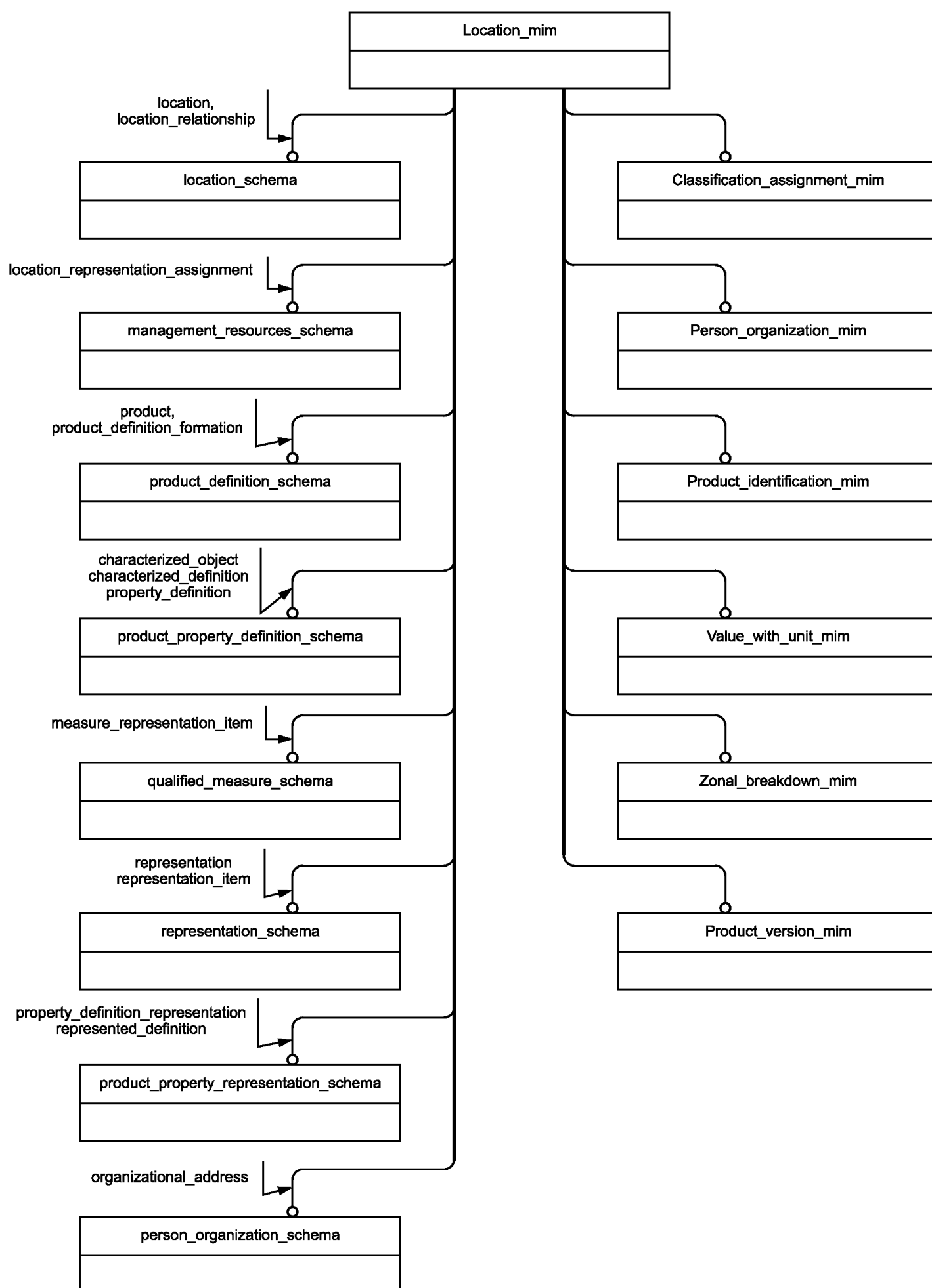
Рисунок D.1 — Представление ИММ на уровне схем в формате EXPRESS-G
