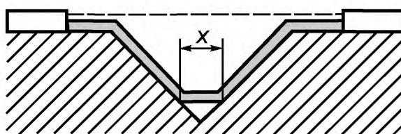
Рисунок Е.3 — Расстояние утечки на примере 2
