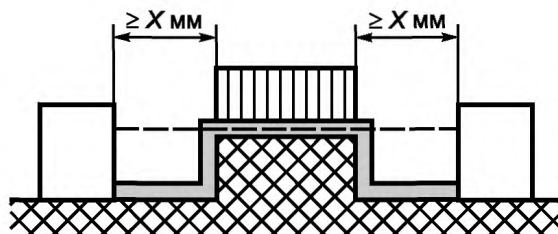
Рисунок E.6 — Расстояние утечки на примере 5
