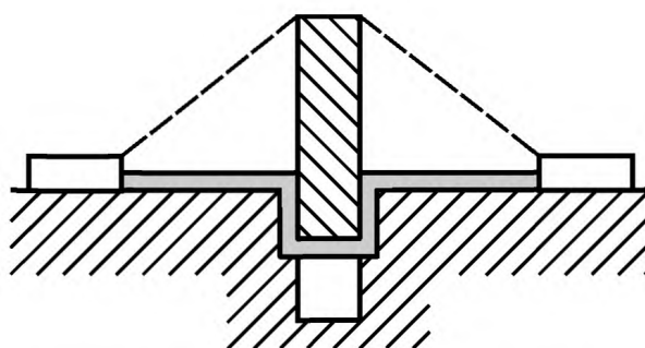
Рисунок E.8 — Расстояние утечки на примере 7
