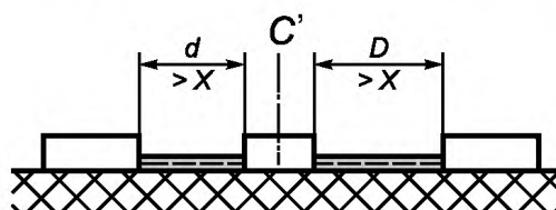
Рисунок Е.11 — Расстояние утечки на примере 10
