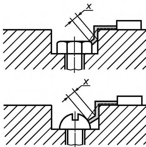
Рисунок Е.10 — Расстояние утечки на примере 9
