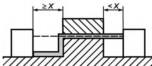
Рисунок E.7 — Расстояние утечки на примере 6
