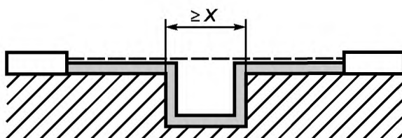
Рисунок Е.2 — Расстояние утечки на примере 1
