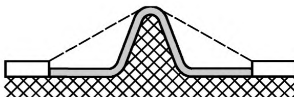
Рисунок Е.4 — Расстояние утечки на примере 3
