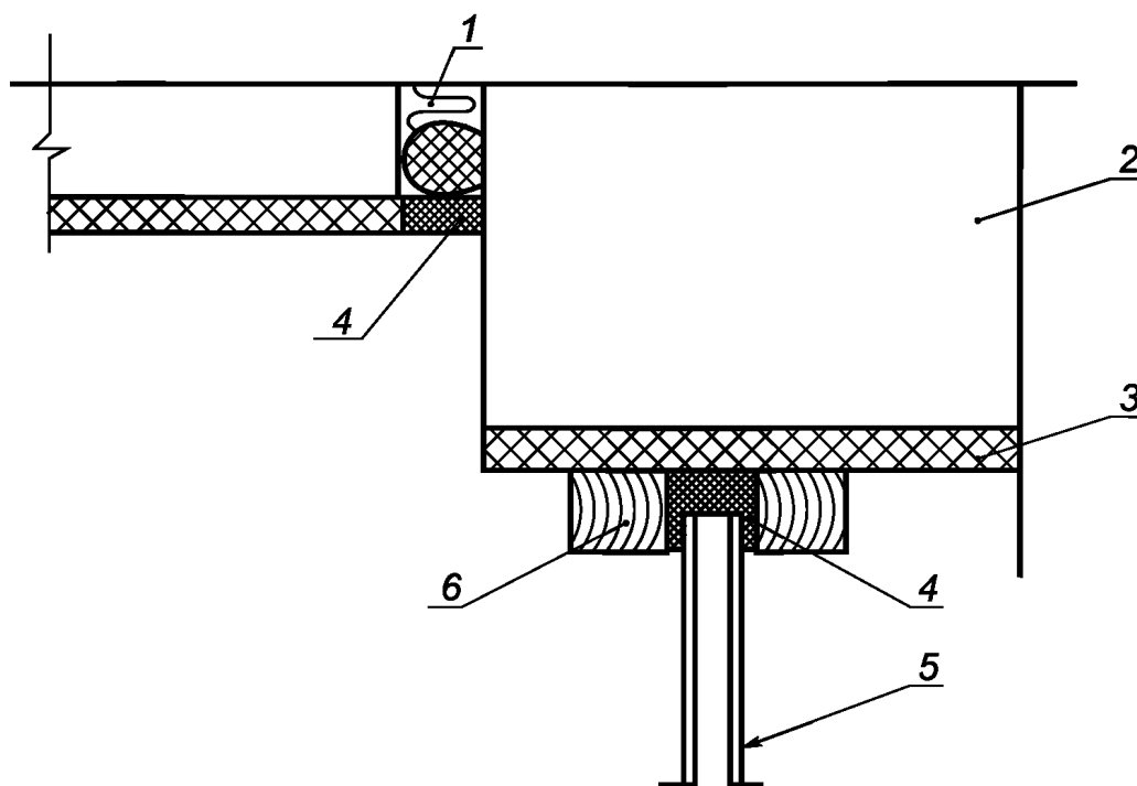
Рисунок 1 — Схема проема между испытательными помещениями высокого и низкого уровней с установленной в нем вспомогательной перегородкой и испытуемым блоком
