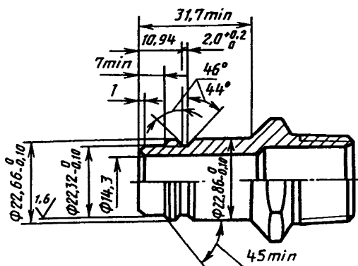
Патрубок для входа охлаждающей воды
