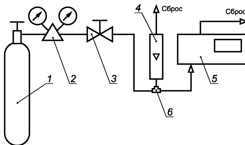
1 — баллон с ГС; 2 — редуктор баллонный; 3 — вентиль точной регулировки; 4 — ротаметр; 5 — СИ наркозных газов; 6 — тройник;
