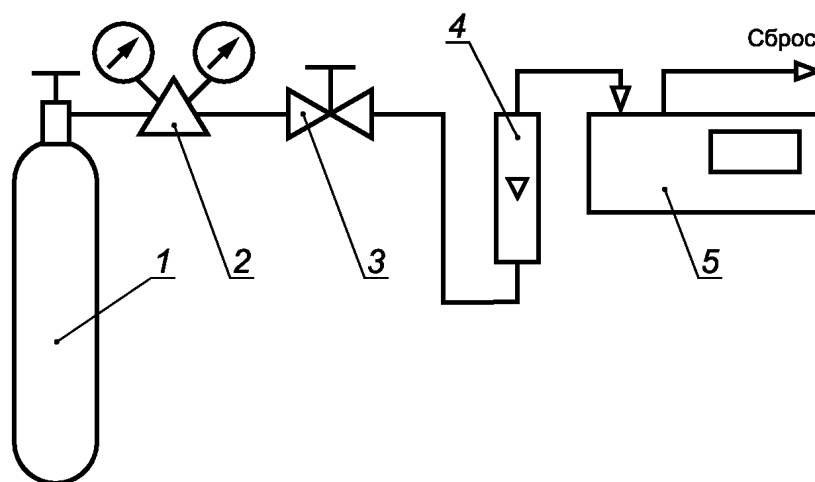
1 — баллон с ГС; 2 — редуктор баллонный; 3 — вентиль точной регулировки; 4 — ротаметр; 5 — СИ наркозных газов
