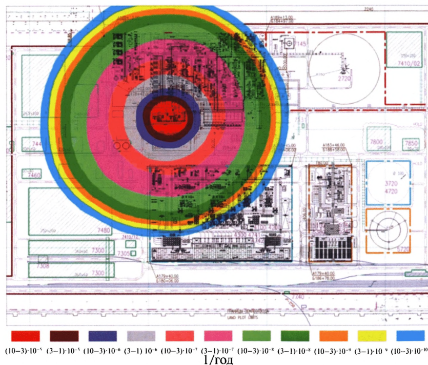
Рис. 5-3. Территориальное распределение потенциального риска разрушения зданий при \Delta P_{\phi} = 28 кПа при авариях на деэтанализаторе со взрывом облака ТВС
