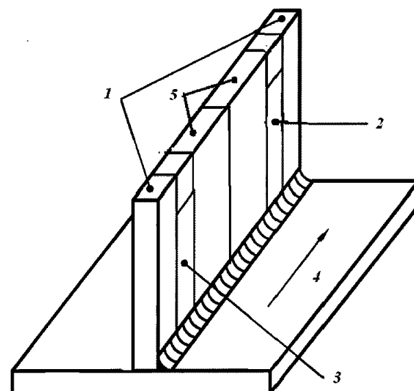
Рис. 6.4.2-3 Схема отбора образцов для механических испытаний от пробы таврового соединения листов угловым швом без разделки кромок:
