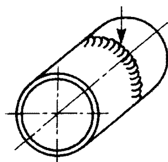
PA: Нижнее положение труба: поворачивается ось: горизонтальная
