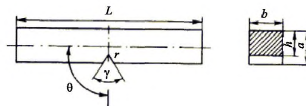
Рис. 6.4.4.2-3 Образец с продольным швом для испытаний на статический изгиб разнородных сварных соединений: А и Б — части пробы из стали различных классов или категорий; L \approx 9a + D — для метода а) или L \approx 11a — для метода б); L — длина образца; a = t ; b = (l_w + 20) мм для t \leq 20 мм и b = (l_w + 30) мм для t > 20 мм
