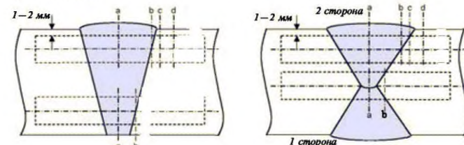
Рис. 6.4.4.4-4 Схема вырезки и расположения надреза на образцах для испытаний на ударный изгиб для технологических процессов сварки сталей высокой прочности:
