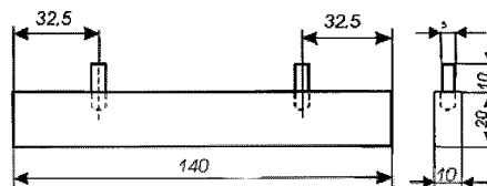
Планка для фиксации зазора
