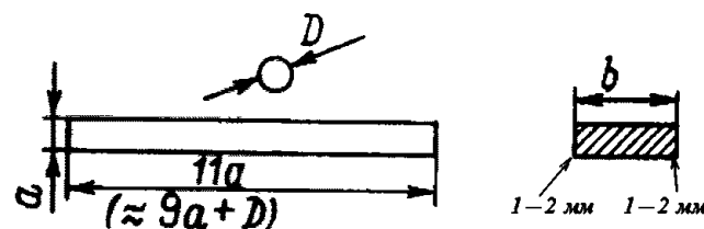
Рис. 6.4.4.2-1 Образцы для испытаний на статический изгиб: а) при t < 12 мм (образцы с растяжением корня и поверхности шва) a = t , b = 30 мм;
