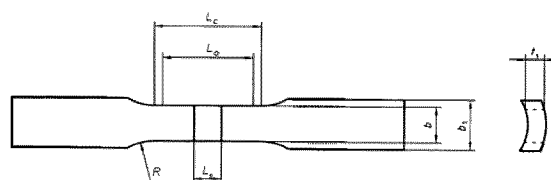
Рис. 6.4.4.1-2 Поперечный образец для испытаний на статическое растяжение из стыкового соединения труб:
