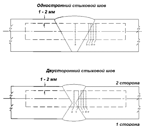
Рис. 6.7.1.5 Схема вырезки и расположения надреза для испытаний на ударный изгиб:
