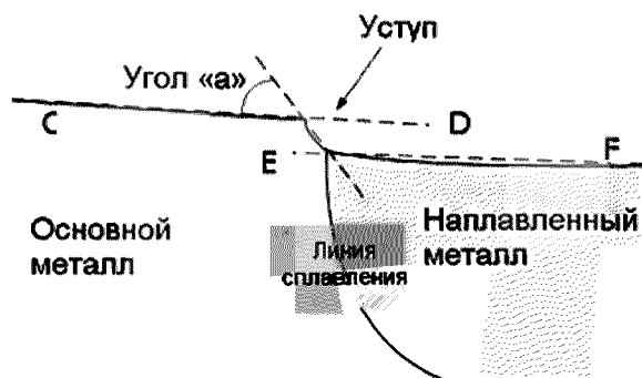
Рис. 2.6.8.3.3.1.1 Определение угла уступа
