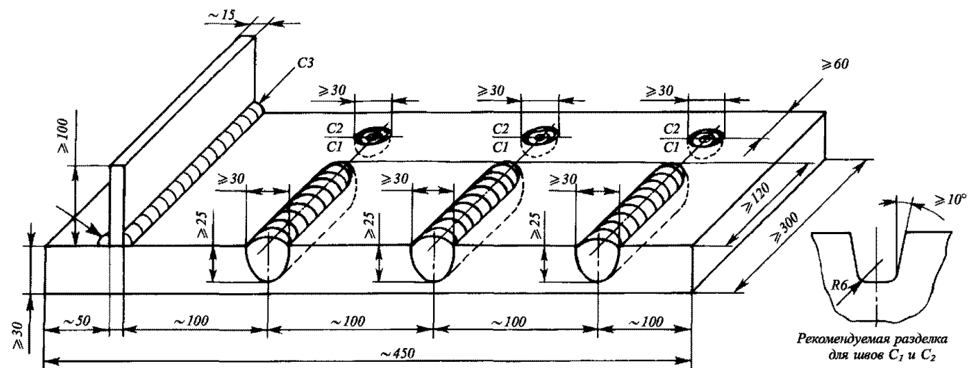
Рис. 8 Проба – имитатор ремонта отливок и поковок Р 8
