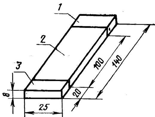
Рис. 5.4.6.2.2 Образец для определения содержания водорода: 1, 3 – выводные планки; 2 – рабочая часть образца (может состоять из нескольких частей равной длины)
