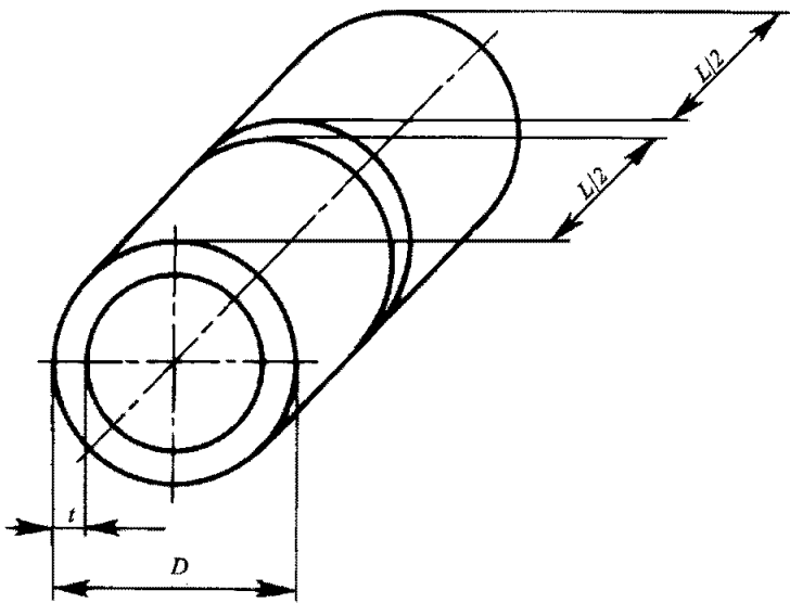
Рис. 3 Проба стыкового соединения труб P 3
