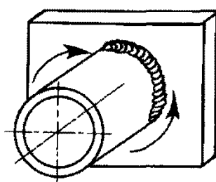
РФ: Вертикальное положение (снизу-вверх) труба: неподвижная ось: горизонтальная
