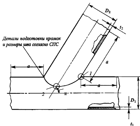
Рис. 7.3.2.4.1 Проба узла сочленения труб/соединения труб угловым швом и схема вырезки образцов: 1 и 2 — места отбора макрошлифов; 1 — место отбора микрошлифа; a \geq 150 мм
