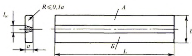
Рис. 6.4.4.2-3 Образец с продольным швом для испытаний на статический изгиб разнородных сварных соединений: А и Б — части пробы из стали различных классов или категорий; L \approx 9a + D — для метода а) или L \approx 11a — для метода б); L — длина образца; a = t ; b = (l_w + 20) мм для t \leq 20 мм и b = (l_w + 30) мм для t > 20 мм
