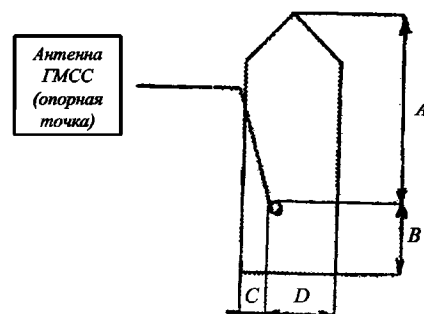
Рис. 5.3 Параметры расположения антенны:
