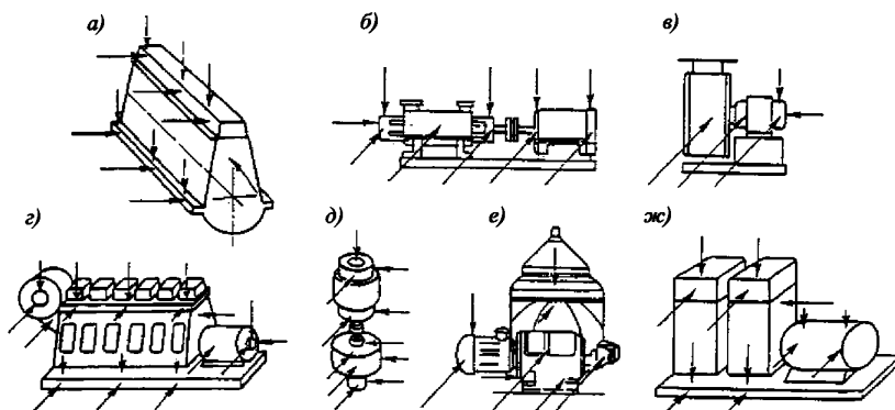
Рис. 2 Точки измерения вибрации:
