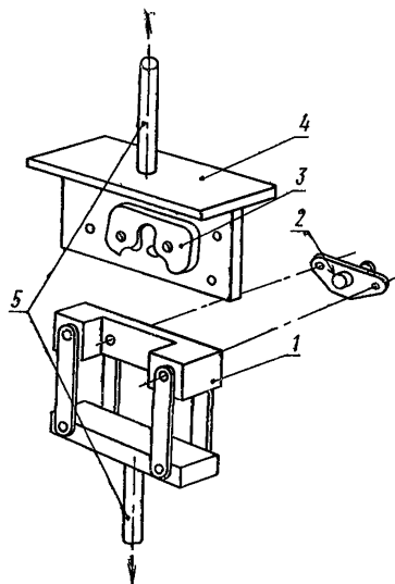
Схема приложения поперечной нагрузки
