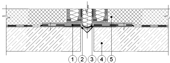
Рисунок 6.5 – Принципиальная схема примыкания в районе деформационном шве
