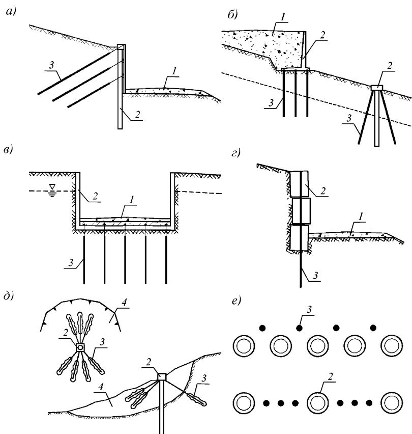
а – анкерное крепление удерживающих сооружений; б – усиление удерживающих сооружений опорными и подкосными микросваями; в – анкерное крепление транспортных сооружений от всплывтия; г – усиление сборных подпорных стен; д – анкерное крепление грунтов склона; е – усиление свайного поля от продавливания грунта; 1 – защищаемый объект, 2 – усиливаемое удерживающее сооружение, 3 – микросваи крепления, 4 – оползневой массив
