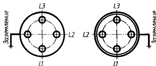
Рис. 16.4.9. Прямое чередование фаз L1 , L2 , L3
