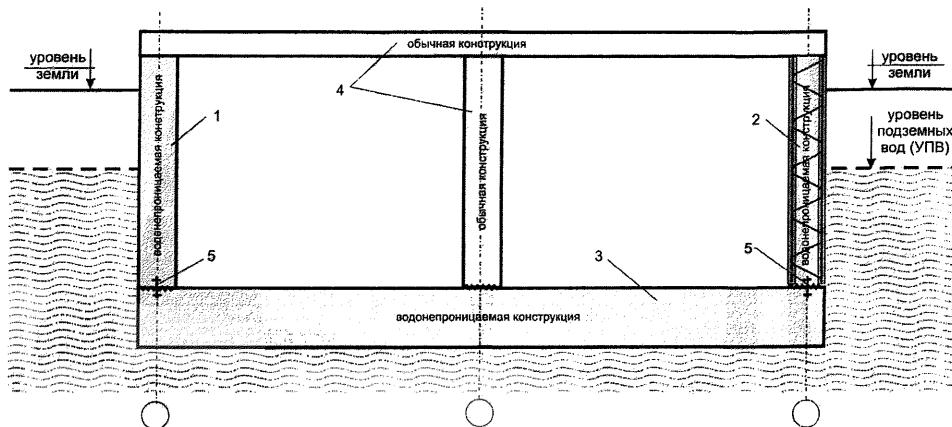
1 — наружная стена (монолитный бетон или сборный элемент); 2 — стеновая система с применением сборных железобетонных элементов несъемной опалубки; 3 — фундаментная плита или ростверк; 4 — перекрытие и внутренняя стена; 5 — рабочие швы с элементами герметизации
