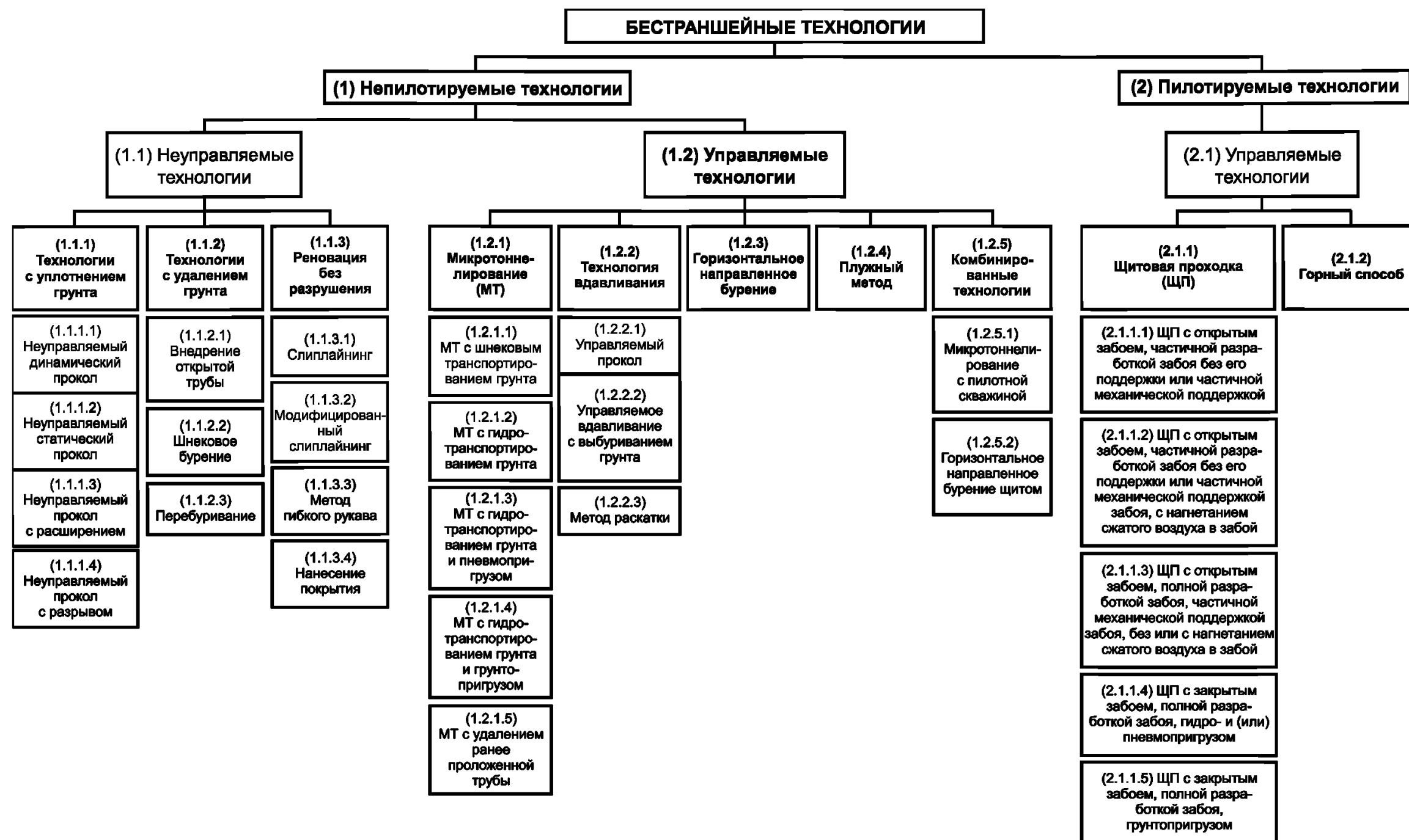
Рисунок Г.1 — Схема классификации бестраншейных технологий
