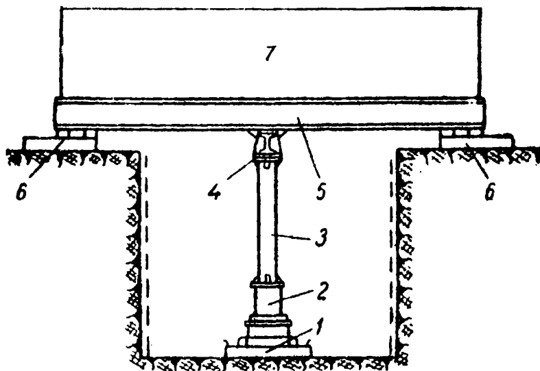
Установка для испытания грунта штампом с упором в грузовую платформу
