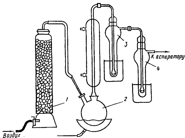
Рис. 1. Схема присоединения приборов: 1 — поглотительная колонка Фрезениуса; 2 — колба с холодильником; 3 — поглотительный прибор, с 10%-ным раствором ацетата свинца; 4 — поглотительный прибор с 1,5%-ным раствором диэтиламина в спирте
