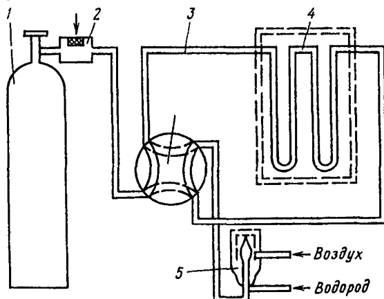
Рис. 2. Схема газового хроматографа с краном обратной продувки:
